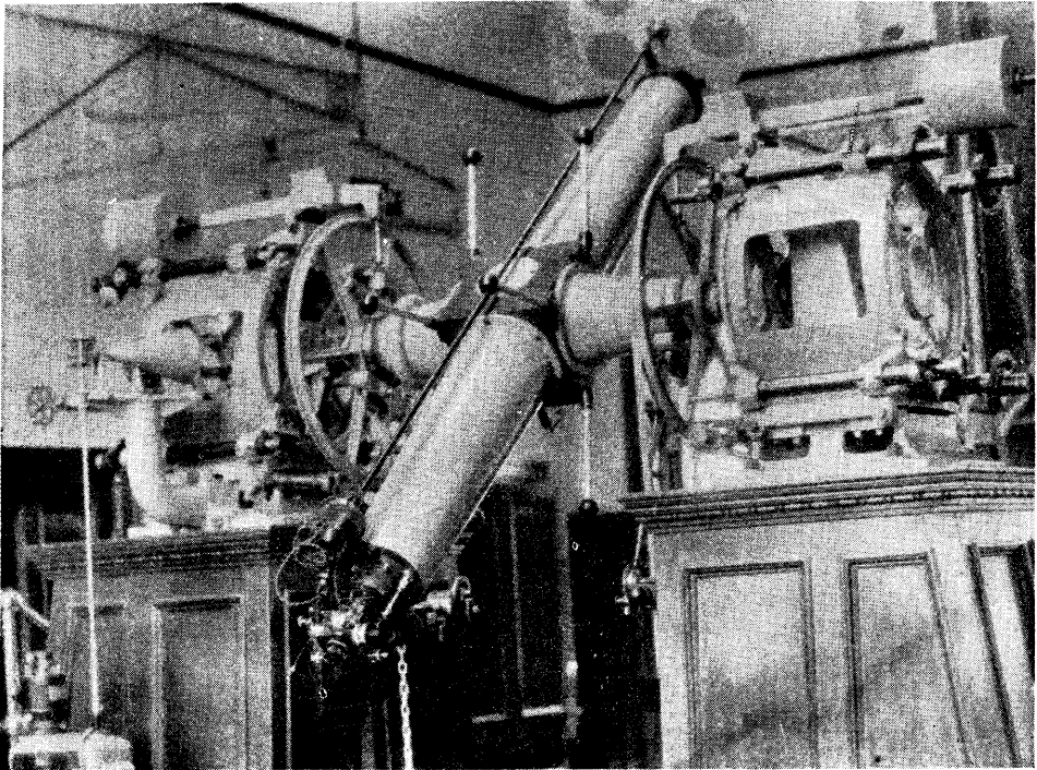
儀午子(圖八第)
