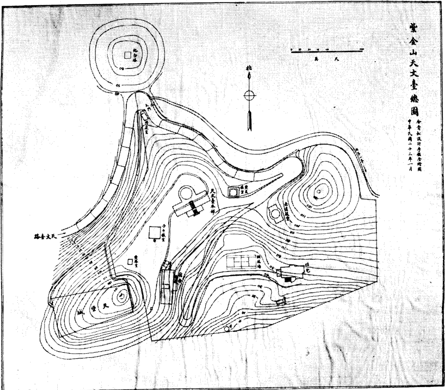
圖 形 地 臺 文 天 (圖 六 第)
