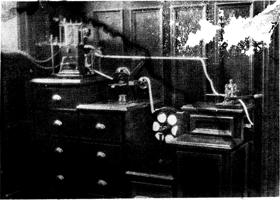
儀時記德利蒲(圖七第)
