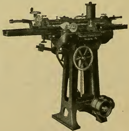
FIG. 106.—TOOL GRINDER.
