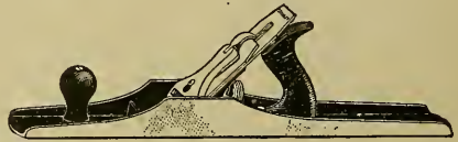
FIG. 31.—JACK PLANE.
