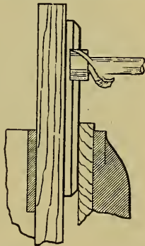
FIG. 221.—ACTION OF A FOSTNER BIT.
