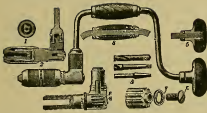
FIG. 211.—A BRACE.
