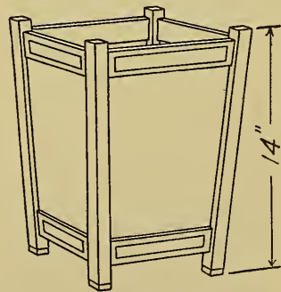
Top 12"X12" Base 10"X10"
