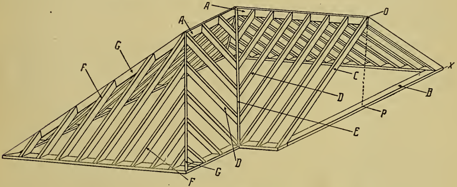
FIG. 179.—ROOF FRAME.
