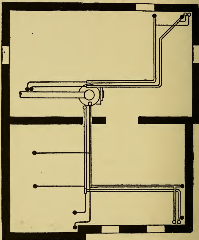
Fig. 76.—Basement.
