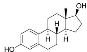
Estradiol.
