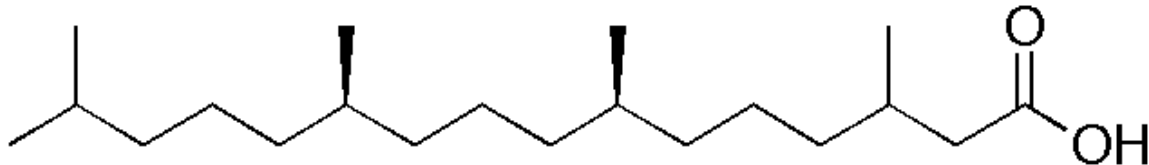
Abb. 464 Phytansäure.
