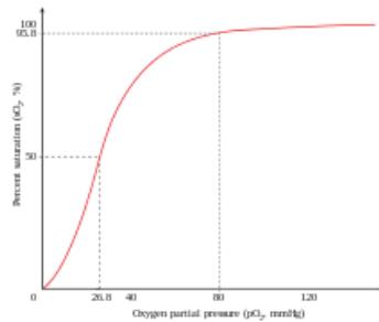
Die Sauerstoffsättigungskurve.
