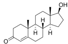
Testosteron.
