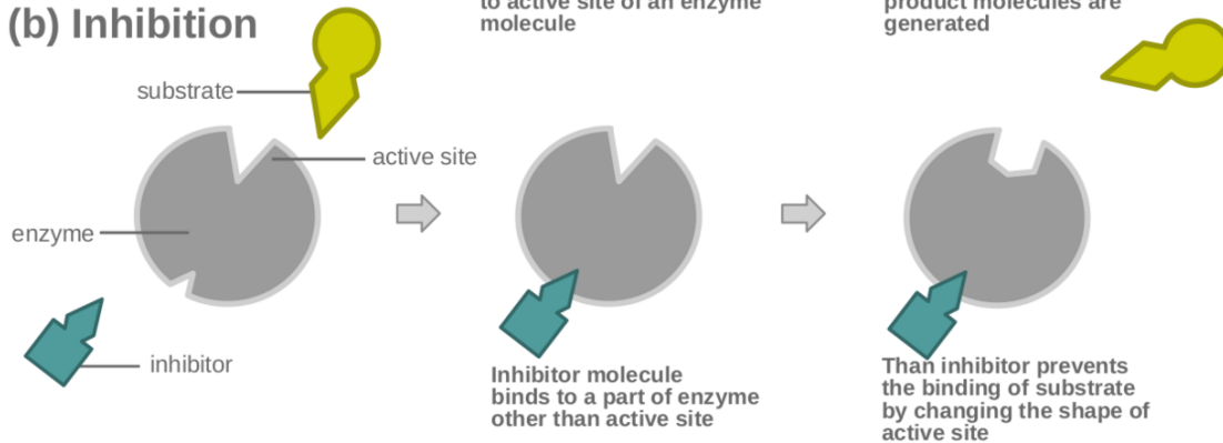
Abb. 8 a) normale Umsetzung b) nicht-kompetitive Hemmung
