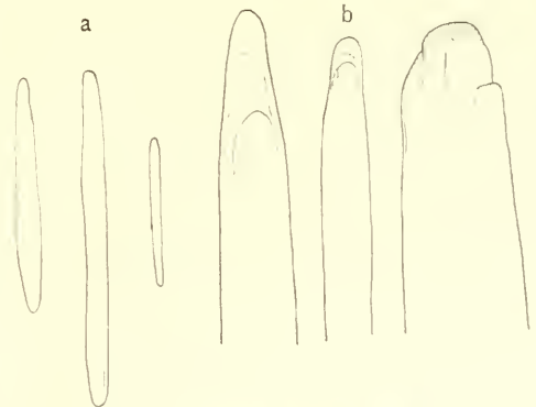
Fig. III. Pteroeides hymenocaulon BLEEKER, Blattspicula; a 3 ganze Spicula, \frac{50}{1} , b 3 Spicula-Endpartien, \frac{240}{1} .
