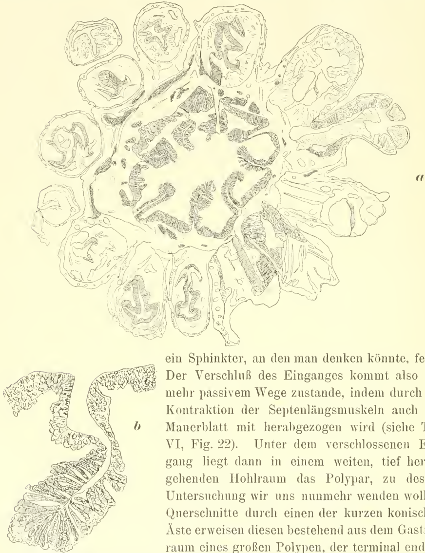
Fig. XLIV. Stuberiotes Semperi (THOMSON). a Querschnitt durch einen Ast; b Teil aus der inneren Partie eines solchen Querschnittes, stärker vergrößert.
