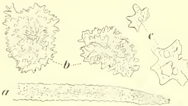
Fig. XXVI. Dendronephthya Michaelseni KÜKTH. var. nov. laevis . Spicula, a aus der Rinde, b aus der unteren Rinde, c aus der unteren Kanalwand.
