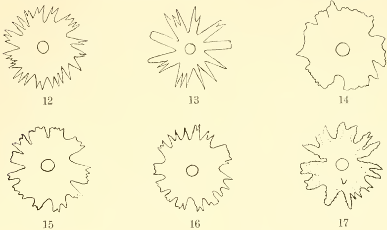
Fig. 12—17. Basale Amphidiskenscheiben; 1125/1 . 12 u. 13 von dem Exemplar der Fig. 11, 14—17 von dem Exemplar der Fig. 10. Fig. 17 eine durch Dörnchen rauhe Scheibe.
