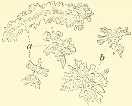
Fig. X. Nephthya Hartmeyerii n. sp. Spicula, a aus der oberen Rinde, b aus der unteren Rinde.
