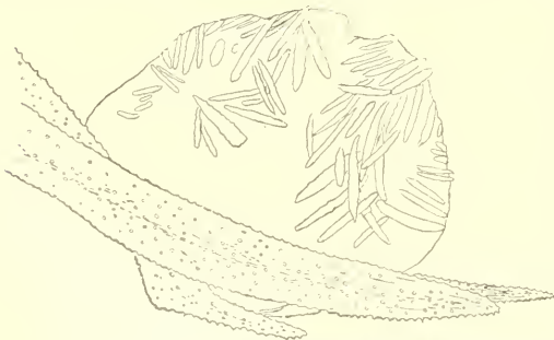
Fig. XXIII. Dendronephthya Michaelсени n. sp. Polyp.
