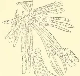
Fig. XXXIII. Nephthyigorgia crassa n. sp. Polyp.
