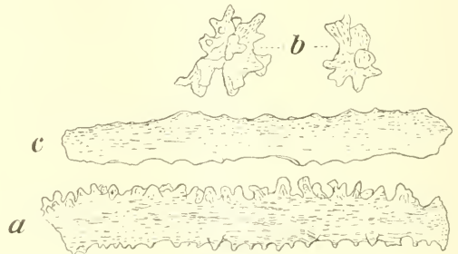
Fig. XVIII. Nephthya australis n. sp. Spicula, a aus der oberen Rinde, b aus der unteren Rinde, c aus der oberen Kanalwand.
