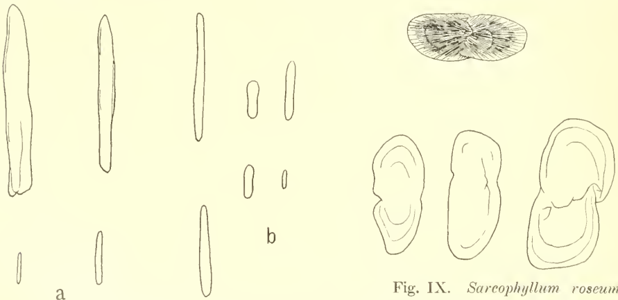
Fig. VIII. Sarcophyllum roseum n. sp., Hautspicula; a aus der Kielhaut, \frac{76}{1} , b aus der Stielhaut, \frac{76}{1} .
