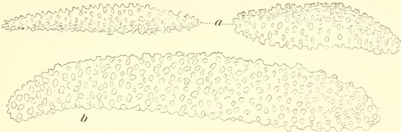
Fig. XXXIV. Nephthyigorgia crassa n. sp. Spicula, a aus dem Kelch, b aus der Kanalwand.
