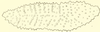
Fig. XVI. Nephthya rubra n. sp. Spiculum aus der Kanalwand.
