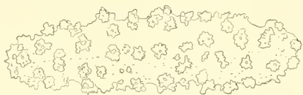
Fig. XXXVIII. Nephthyyigorgia aurantiaca n. sp. Spiculum aus der unteren Rinde.
