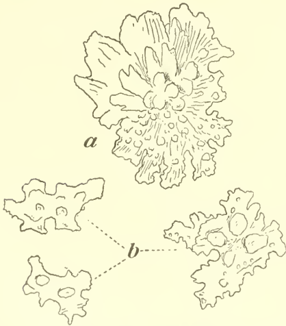
Fig. 1. Plexaurioides filiformis KÜKENTH. Spicula, a aus der obersten Schicht des Cönenchymys, b aus der tieferen Schicht der Rinde.
