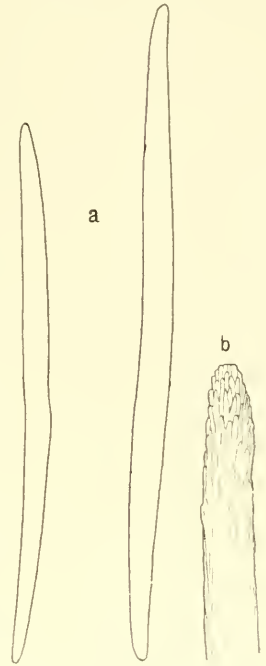
Fig. II. Pteroeides hymenocaulon BLEEKER. Nadeln der Hauptstrahlen; a zwei ganze Nadeln, \frac{15}{1} , b Nadelende, \frac{50}{1} .
