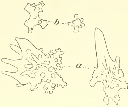
Fig. XLVII. Plexauroides Michaelsoni KÜKTH. Spicula, a aus dem Cönenchym, b aus der tieferen Rinde.
