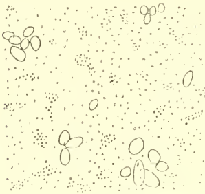
Fig. IV. Pteroeides hymenocaulon BLEEKER, Spicula der inneren Stielschicht, 370/1 .
