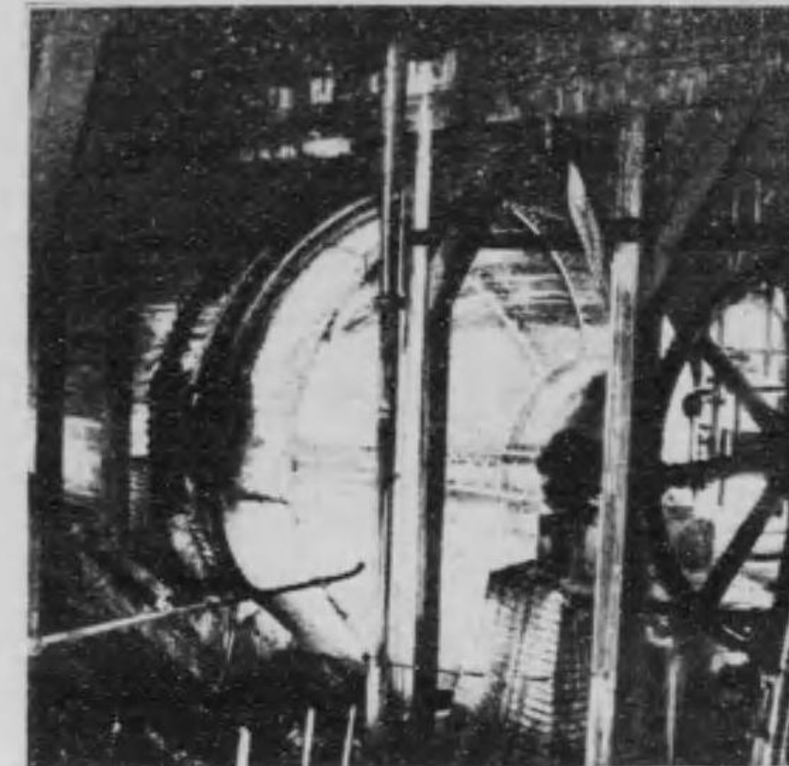
1. 蒸煮釜 (原料とアルカリをいれ水蒸氣を通じつゝ回轉す)
