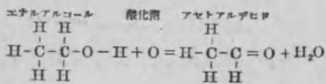
第174圖一熱したる白金の接觸作用により、アルコールをアルデヒドに變ず。
