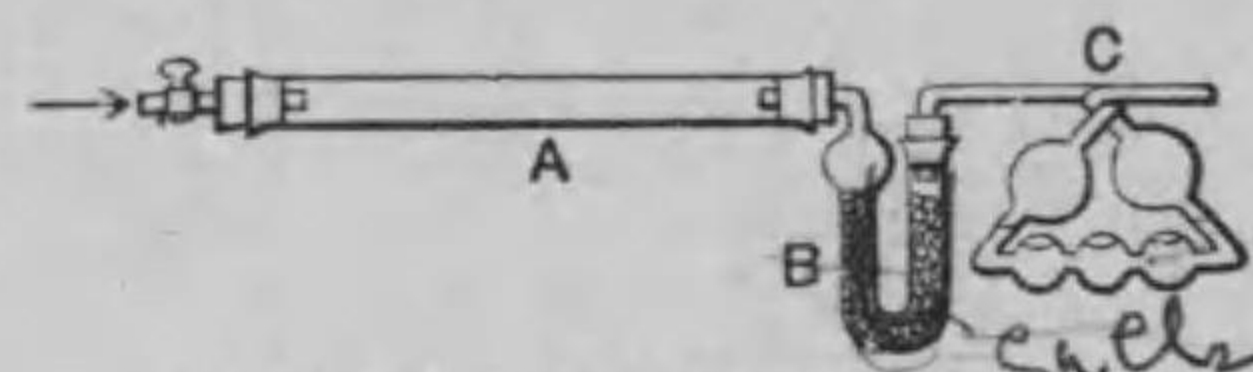
第172圖—有機化合物の定量装置。
