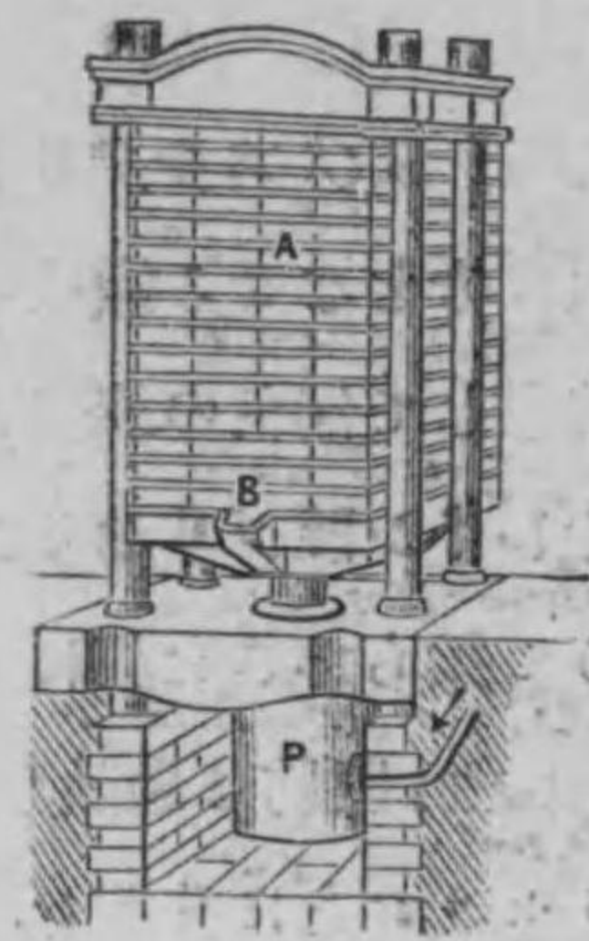
第183圖—植物の子實を押し油を搾る。 (A) 子實壓搾板、(B) 油口、 (P) 水壓機。
