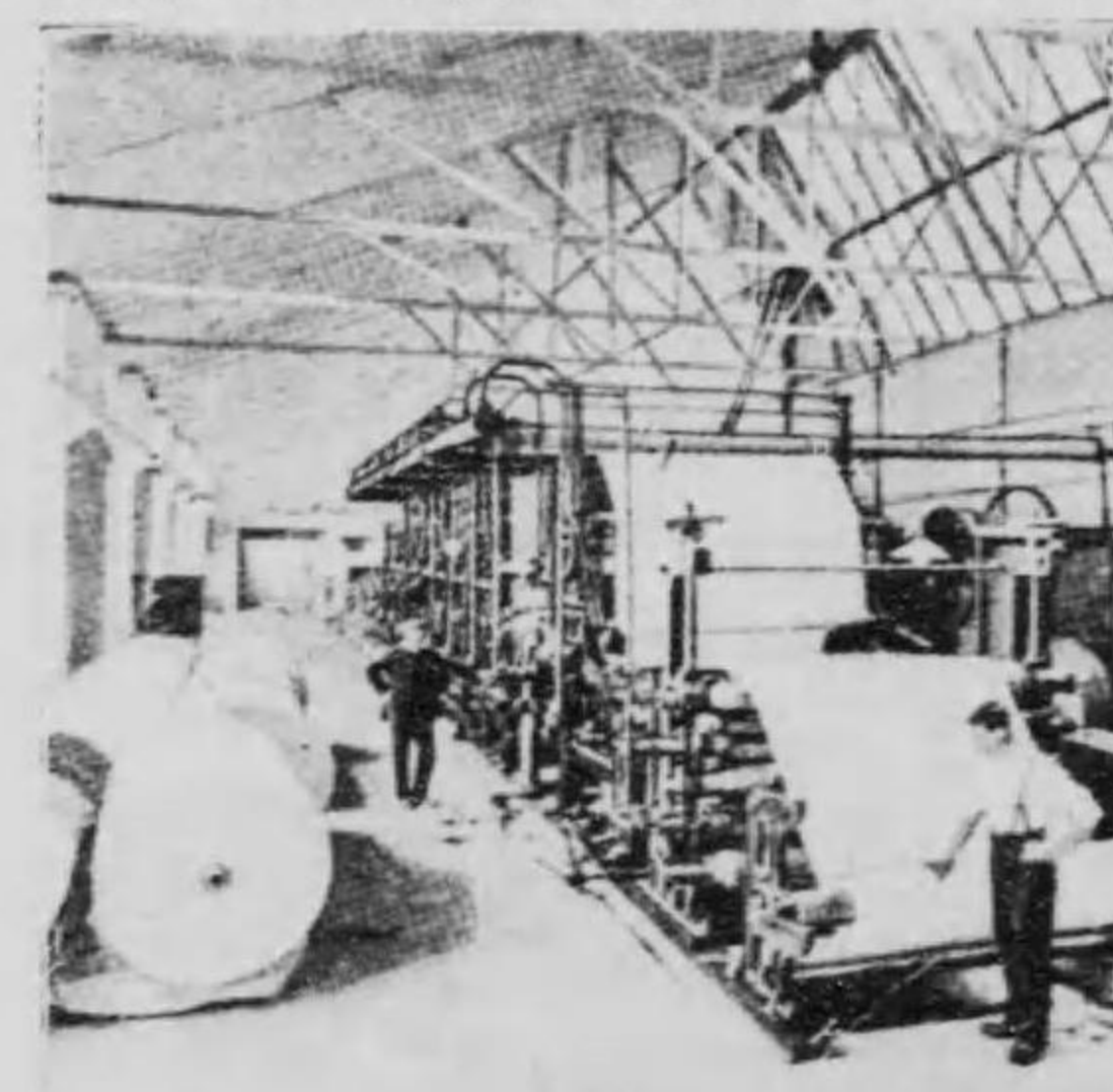
6. 抄紙機(後部) (乾きたる紙を捲く) (612頁參照)
