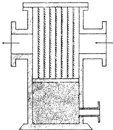
FIG. 7. Condenser.
