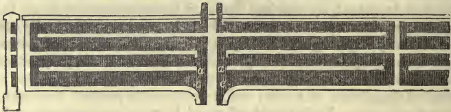
Fig. 121. Longitudinal section of a flued wall.
