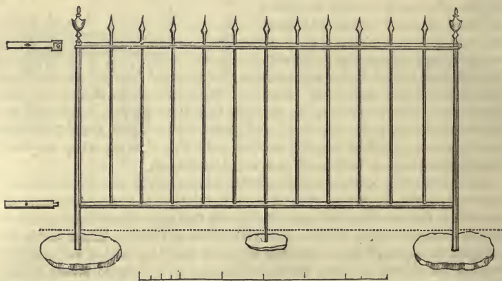
Fig. 333. Cast-iron Espalier-rail.
