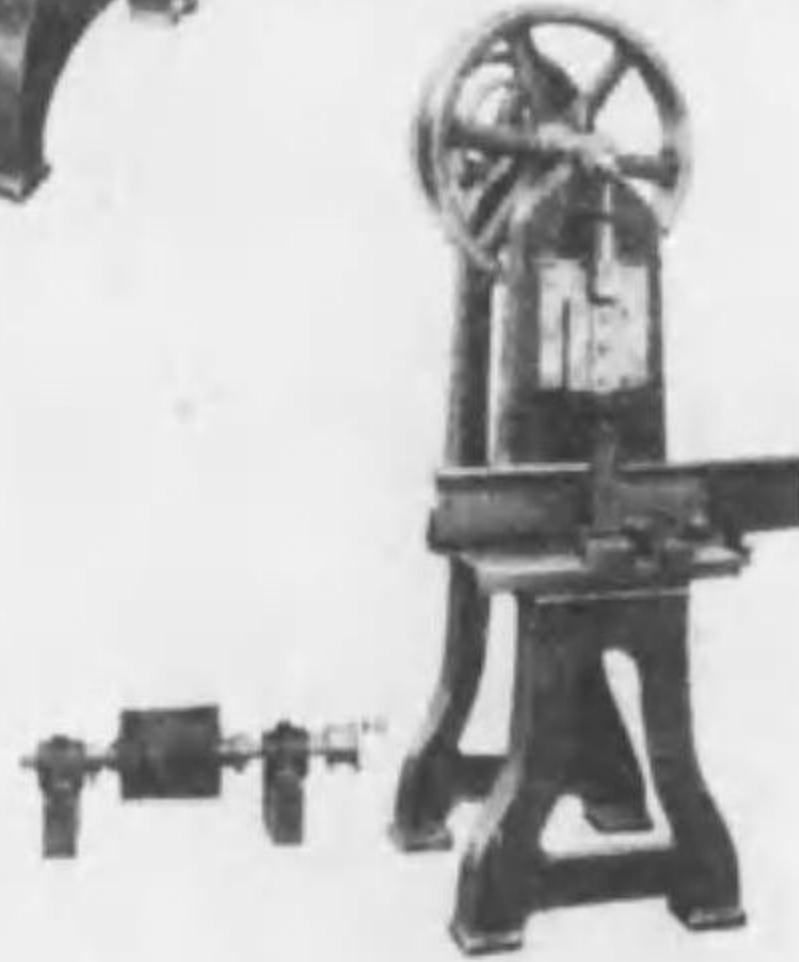
國策型 再生古箴解體機
