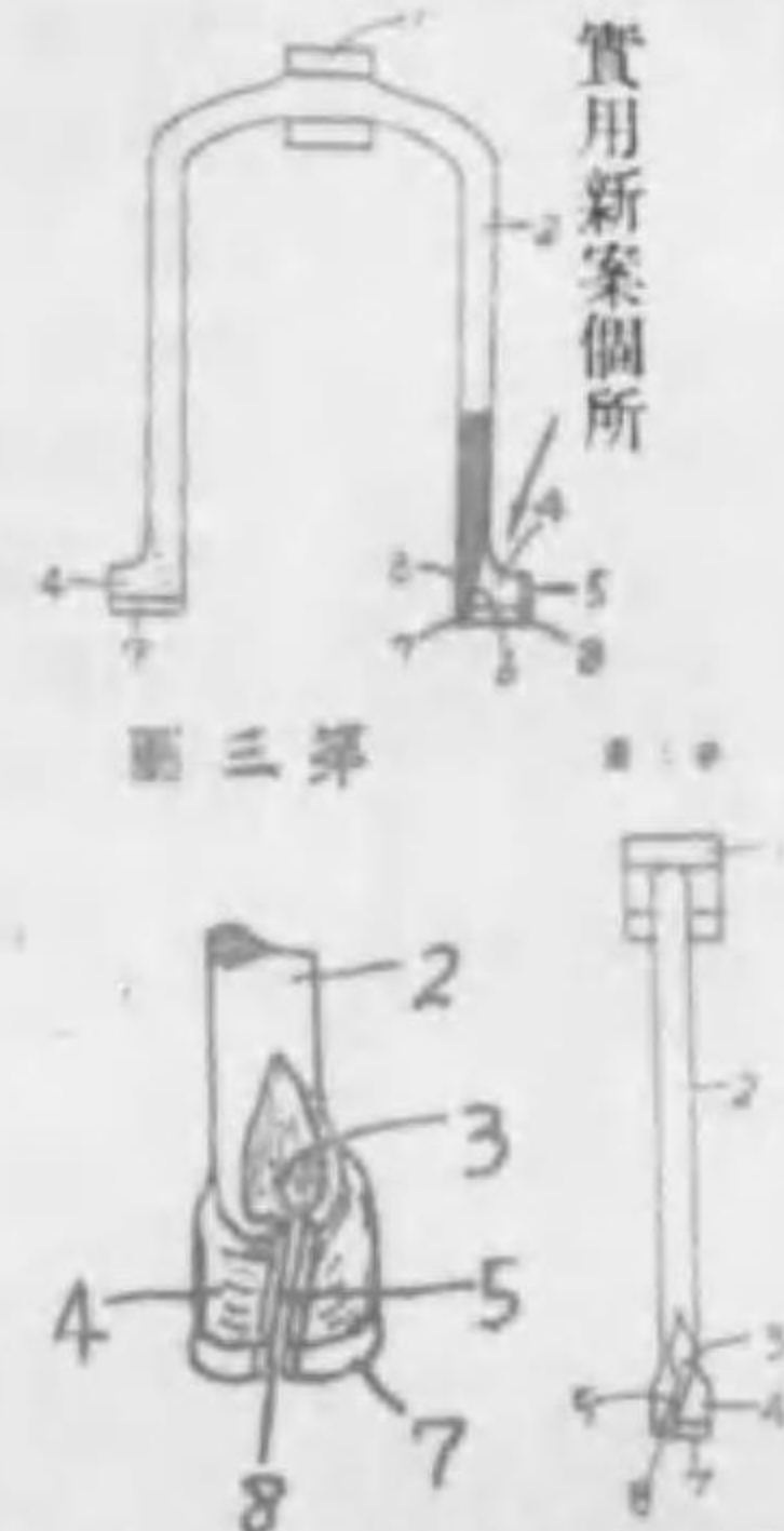
實用新案麻糸用フライヤー
