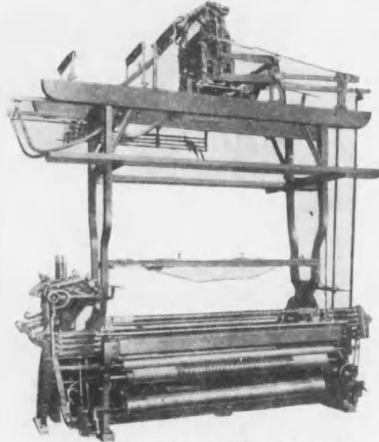
兩口式上下一方ダブルシンダージャカード機
