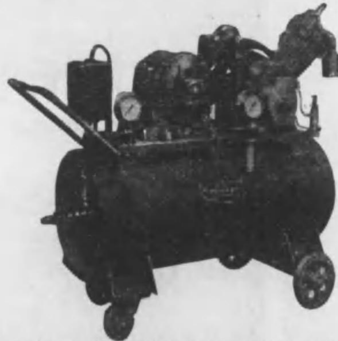
特許AC-IA型可搬式空冷二段空氣壓搾機
