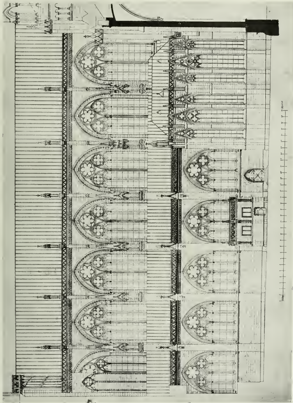
AUFRISS DES LANGHAUSES - SÜDSEITE
