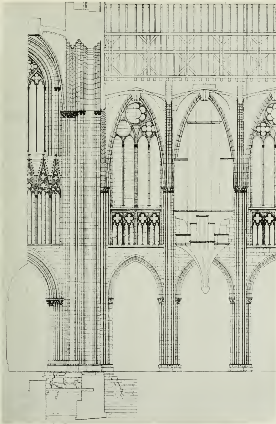
TEIL DES LÄNGSSCHNITTS - TURMJOCH UND LANGHAUSJOCH
