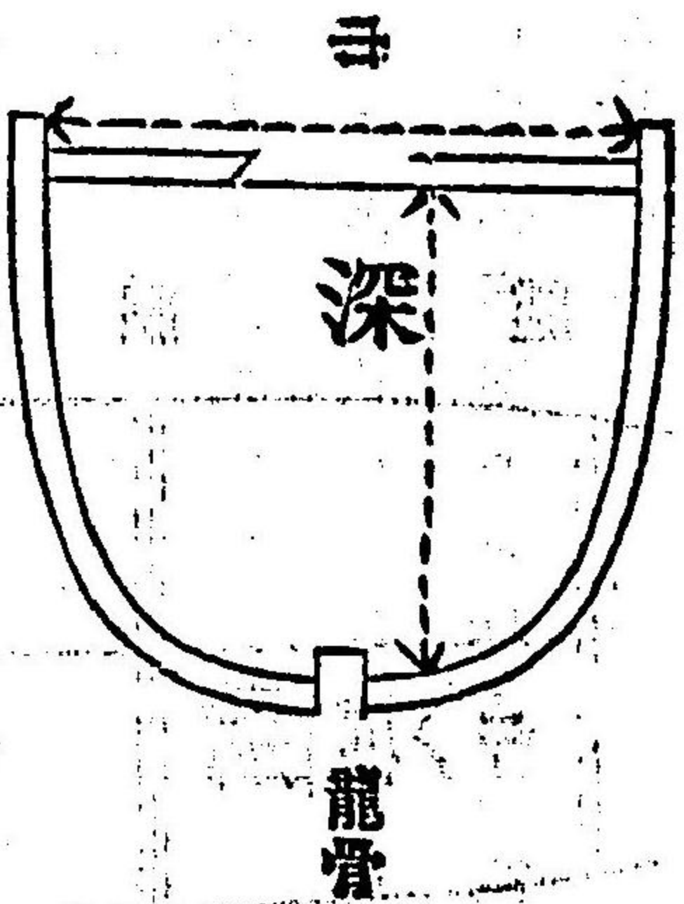
船ノ胴正面
