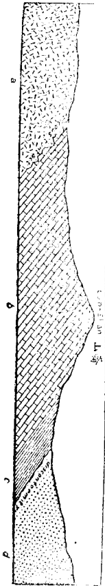
第十三圖 南京附近崙山石灰岩層
