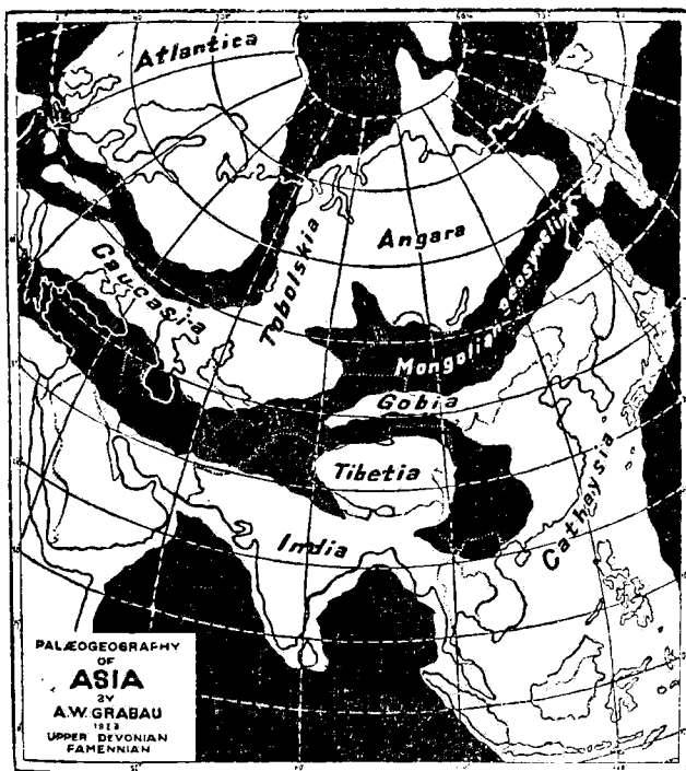
第二十圖 第十七圖之後期
