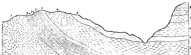
第八圖 雲南東部之寒武系
