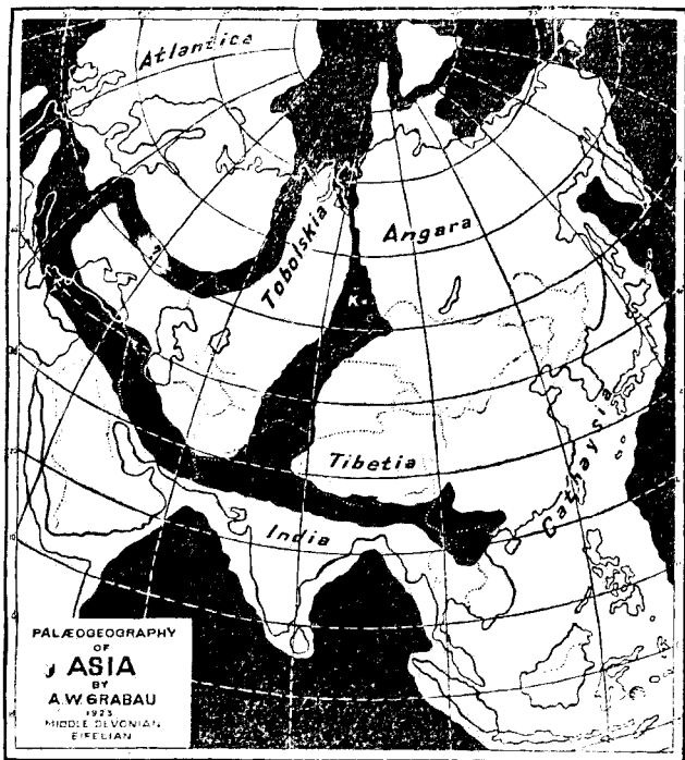
第十六圖 中部泥盆紀時代亞洲水陸分布狀況
