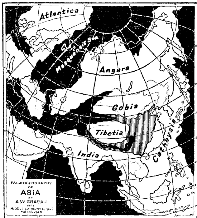
第二十三圖 莫斯科層時代亞洲水陸分布狀況
