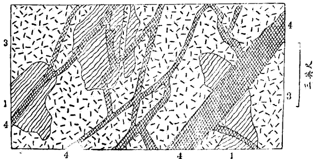
第二圖 泰山系局部的擴大
