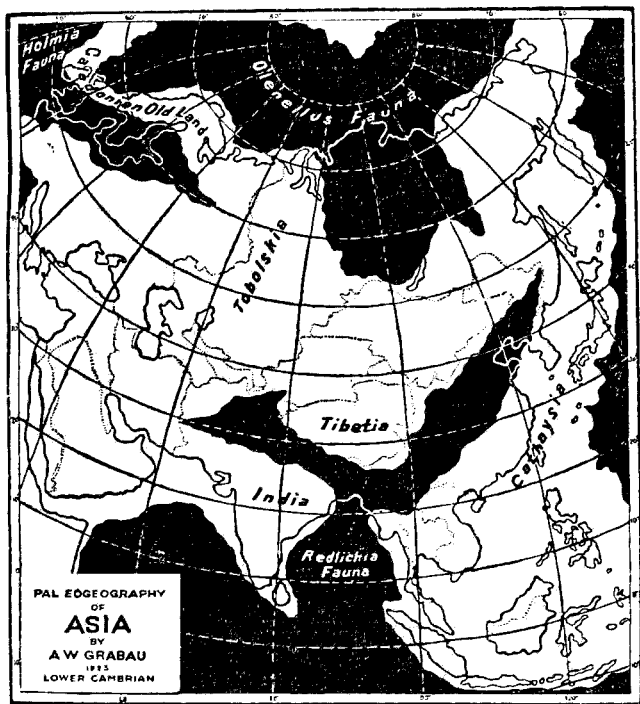
第五圖 下部寒武紀時代亞洲之水陸分布狀況
