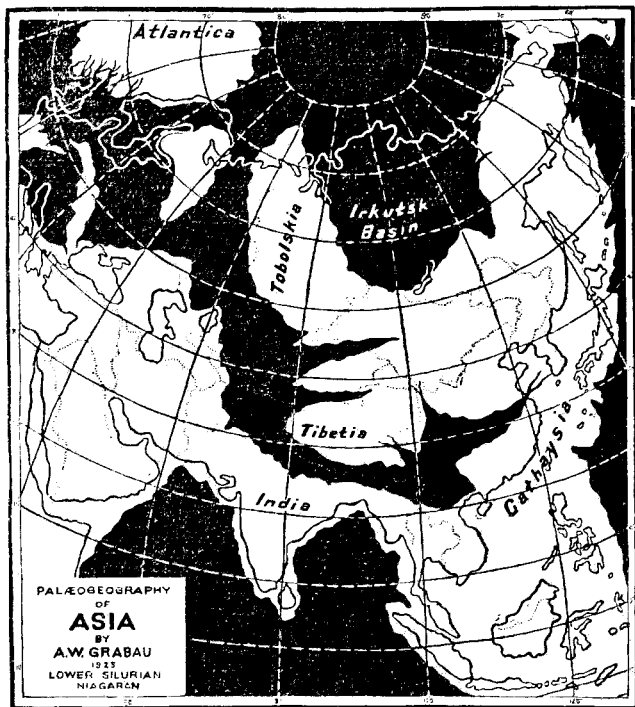
第十四圖 下部志留紀時代亞洲水陸分布狀況
