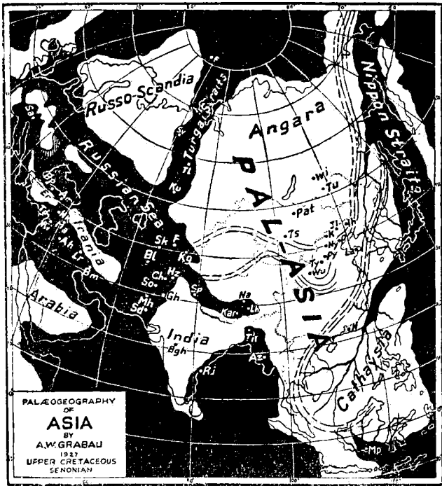
第二十九圖 上部白堊紀亞洲海陸分布狀況
