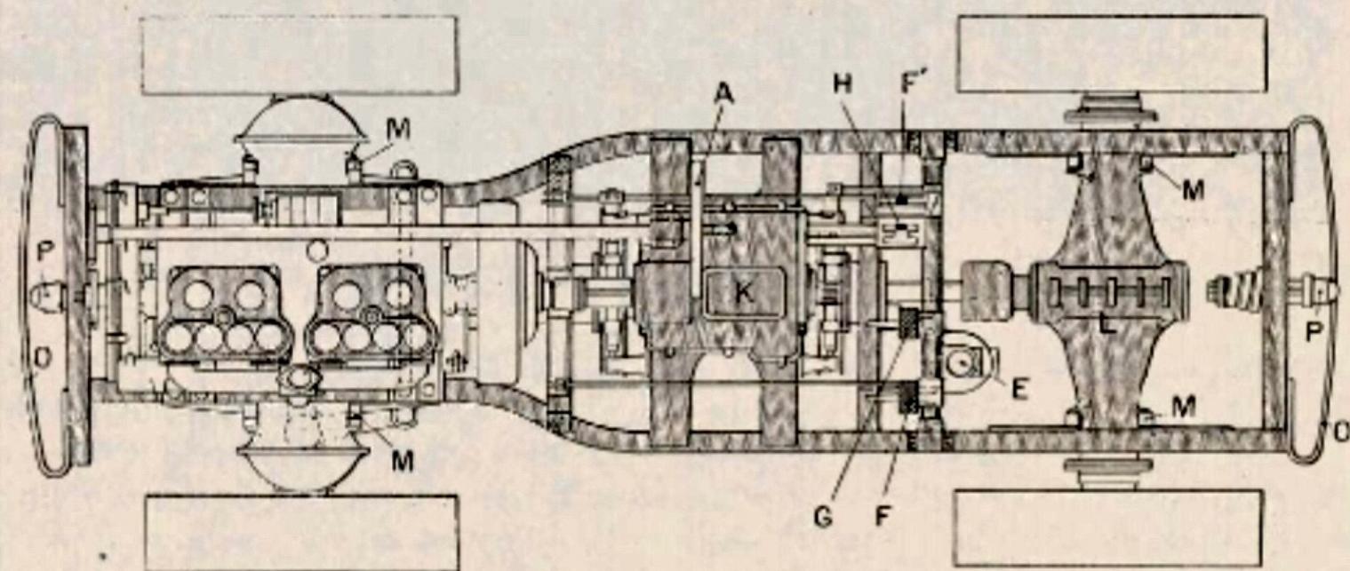
Fig. II. — ÉLÉVATION ET PLAN DU TRACTEUR WILFORD. — A, volant de mise en marche du moteur. — B, ventilateur commandé par le moteur. — C, réservoir à eau et radiateur. — E direction. — F, pédale de frein. — F', levier de frein. — G, pédale de débrayage. — H, commande de changement de vitesse. — J, transmission à cardan. — K, boîte des vitesses. — L, carters des vis sans fin de transmission et des différentiels. — M, plaques de garde des roues. — N, plaques de garde avant et arrière. — O, tampons. — P, crochets d'attelage.
