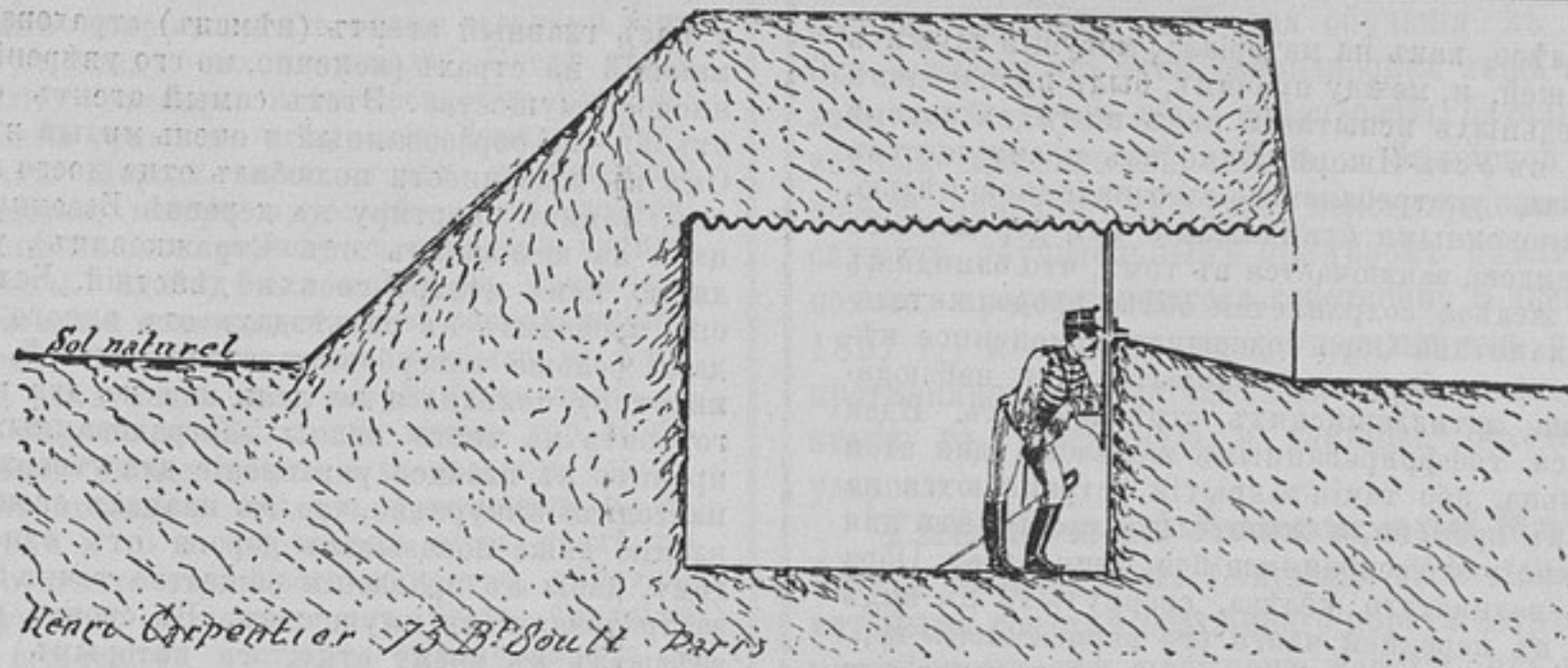
Разрѣзь блиндажа изъ гофрированного желѣза.
