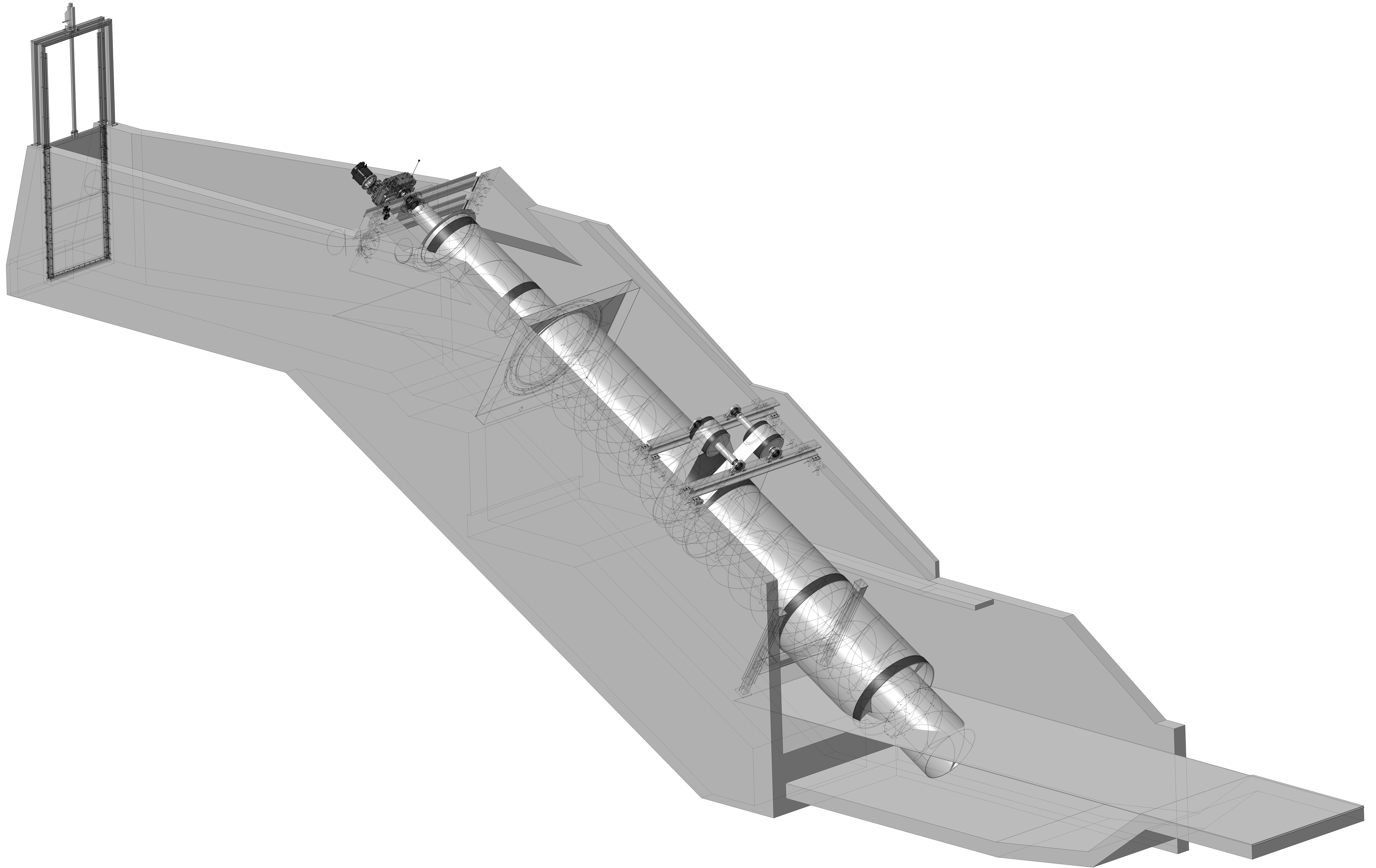
Isometrische Ansicht Maßstab: 1:25
