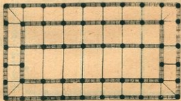
殿閣地盤殿身七間副階 周匝各兩架椽身內單槽
