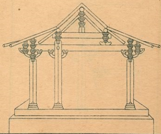
四架椽屋對牽二椽椽用三柱
