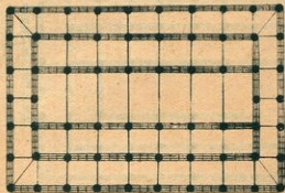
殿閣地盤殿身七間副階 周匝各兩架椽身內雙槽
