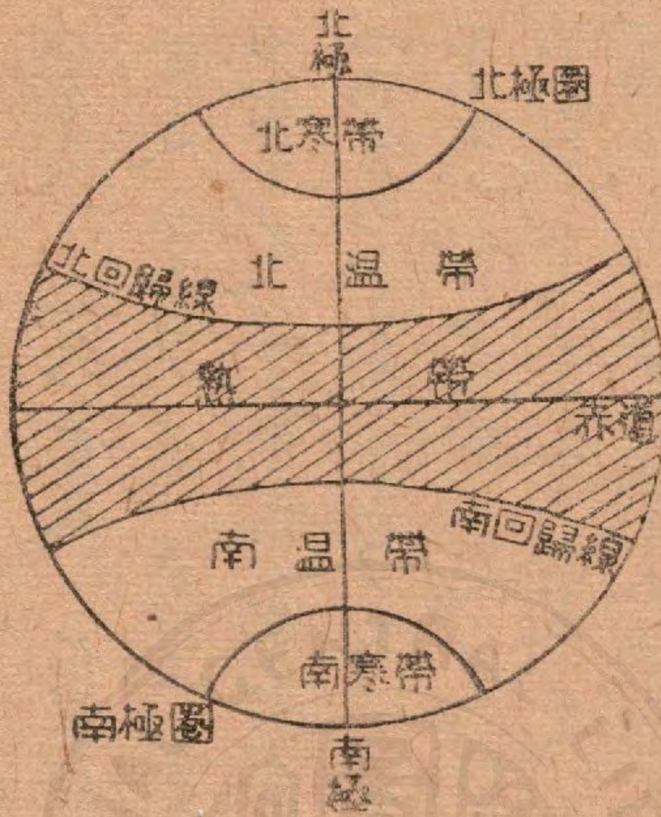
地球五帶圖
