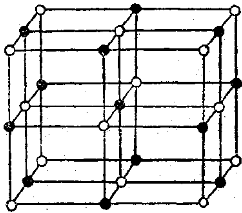
ClNa. 體晶結的鹽食
