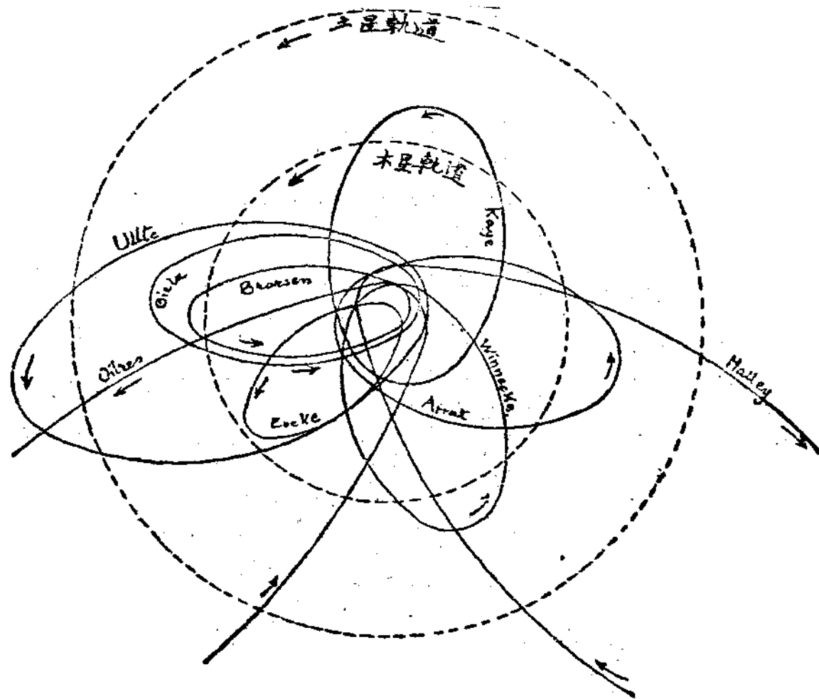
（道軌的星彗）五圖
