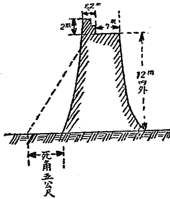
(側 斷 面)
