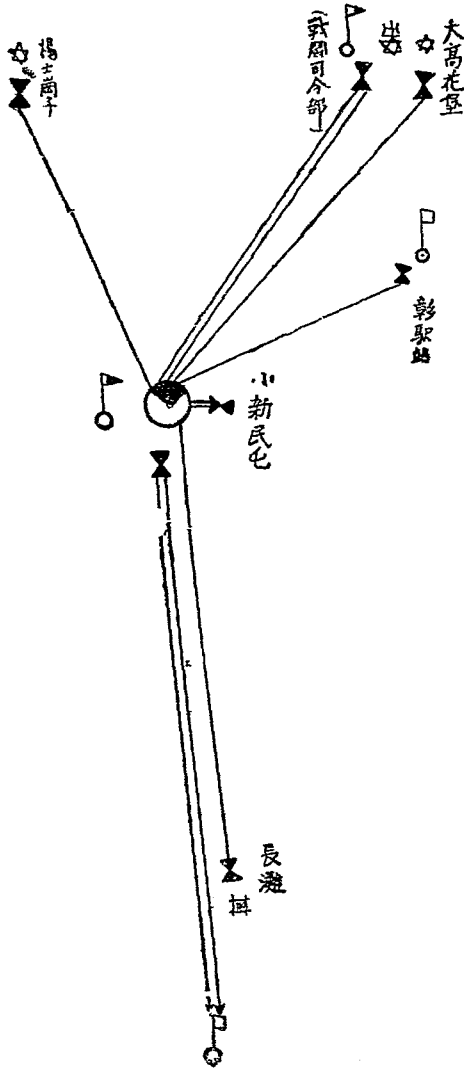
第十師有線通信網之線要圖 二十七日拂曉
