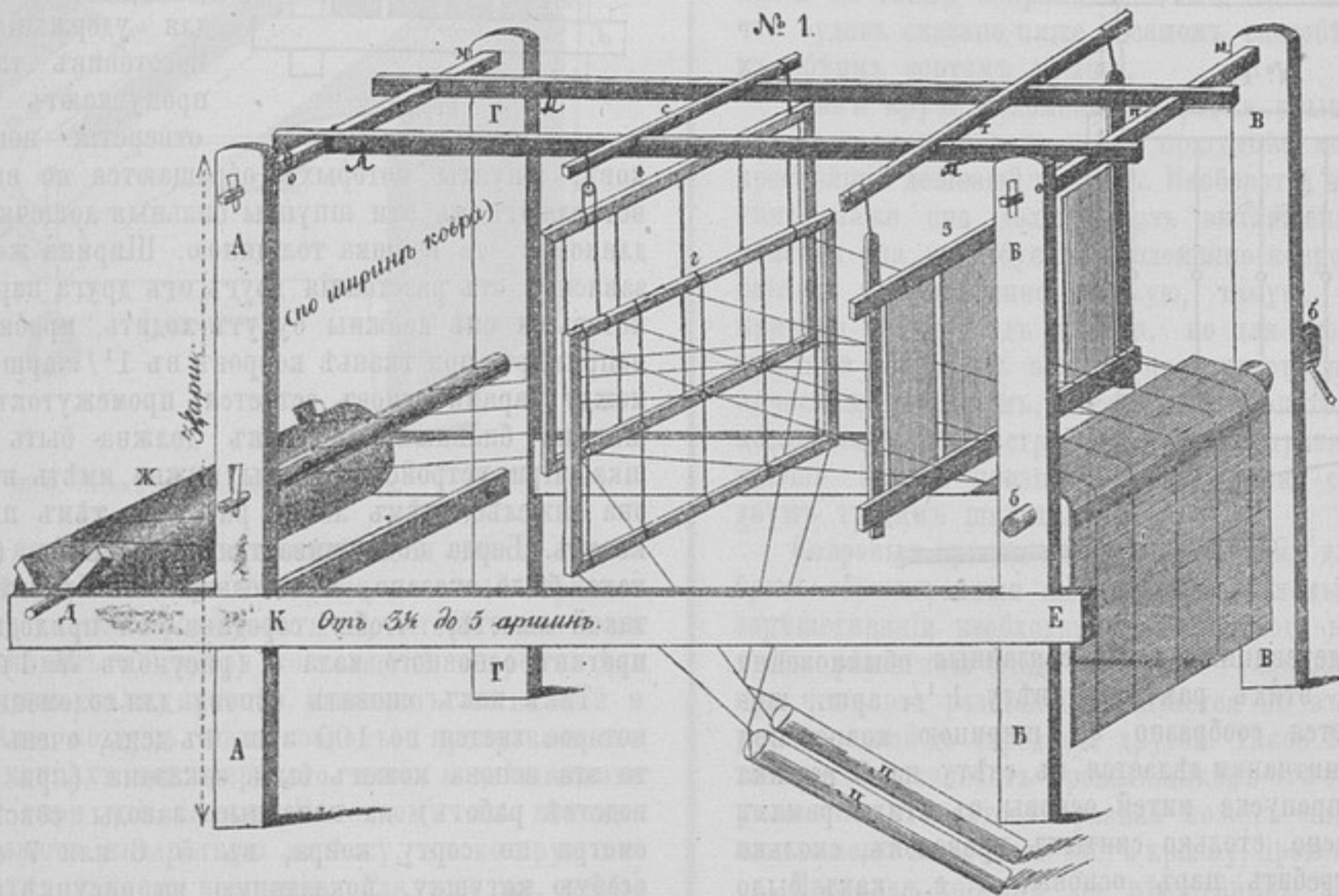
Ткацкій станокъ.
