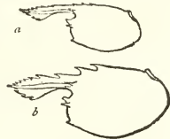
FIG. 27. Spirontocaris dalli (× 2½). Attu.
