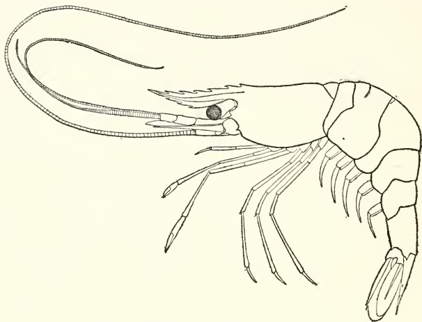
FIG. 9. Palæmonetes kadiakensis . ♀ (× 2½). Kadiak.
