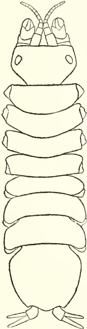
FIG. 102. Janiropsis kincaidi sp. nov. ( \times 27 ).
