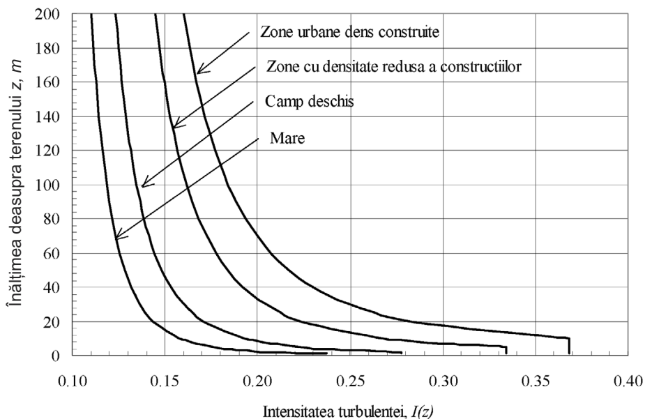
Fig. 3. Intensitatea turbulenței I(z)
