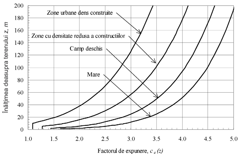
Fig. 5. Factorul de expunere, c_e(z)
