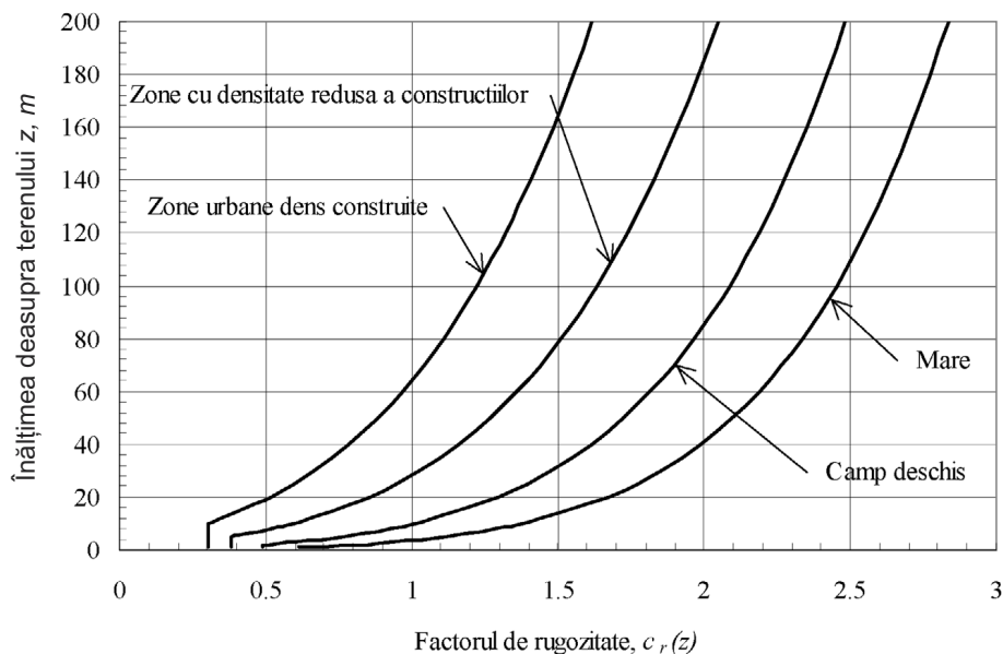
Fig. 1. Factorul de rugozitate, c_r(z)
