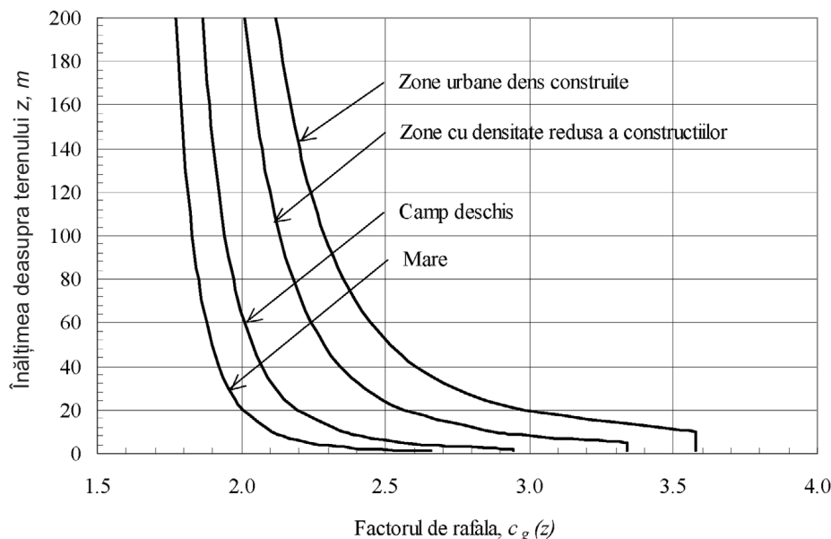
Fig. 1. Factorul de rafală, c_g(z)
