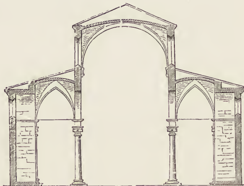
Fig. 128. Servi zu Siena. Querschnitt. (L.)
