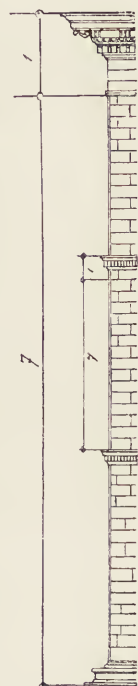
Fig. 58. Vom Pal. Strozzi zu Florenz. (Nach A. Thiersch.)
