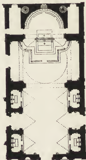
Fig. 138. S. Maria de' Monti. (Nach Letarouilly.)
