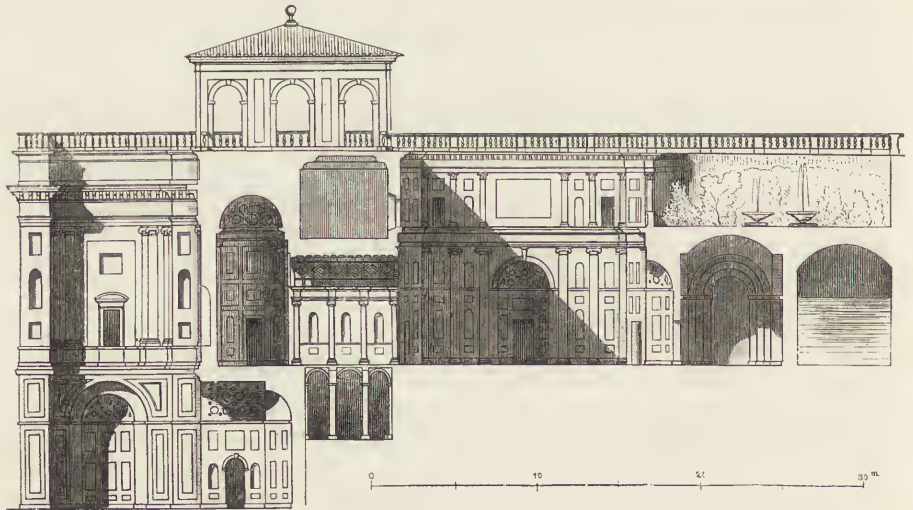
Fig. 231. Monte Imperiale bei Pesaro. (Fig. 228—230 aus dem Archiv des Municipio von Pesaro, mitgeteilt durch H. Herdtle.)
