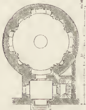
Fig. 100. Capp. Pellegrini in S. Bernardino zu Verona.
