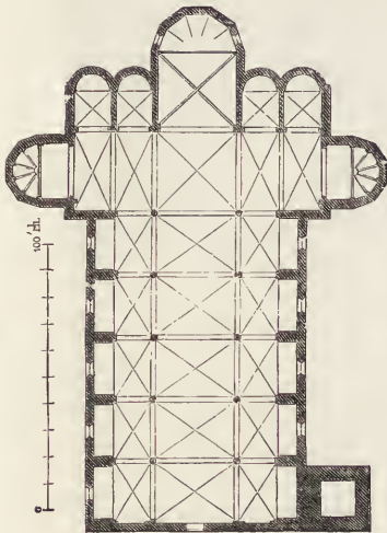
Fig. 127. Servi zu Siena. Grundriss. (L.)
