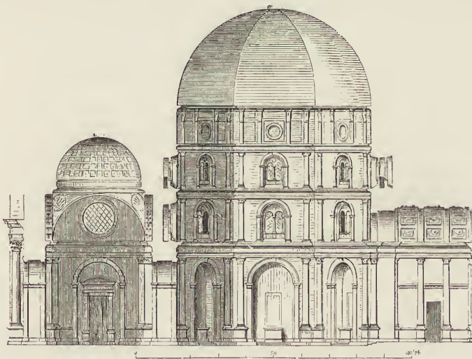
Fig. 83. Madonna dell' Umiltà zu Pistoja. Durchschnitt. (J. Stadler.)
