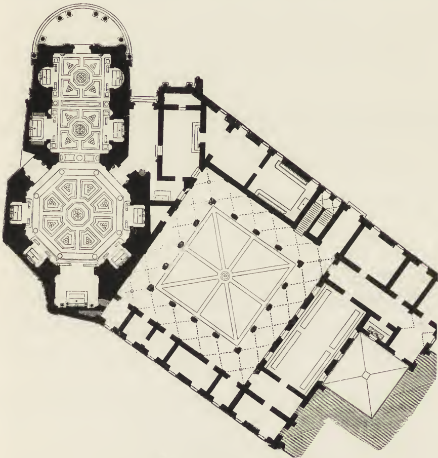
Fig. 162. S. Maria della Pace. (Nach Letarouilly.)
