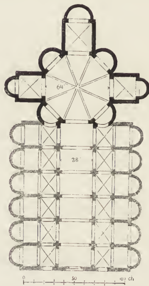
Fig. 104. S. Maria della Passione zu Mailand.
