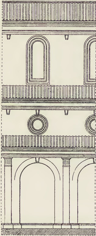
Fig. 161. S. Lorenzo in Florenz. Theilaufriß der Langseiten. (Nach Bühlmann.)
