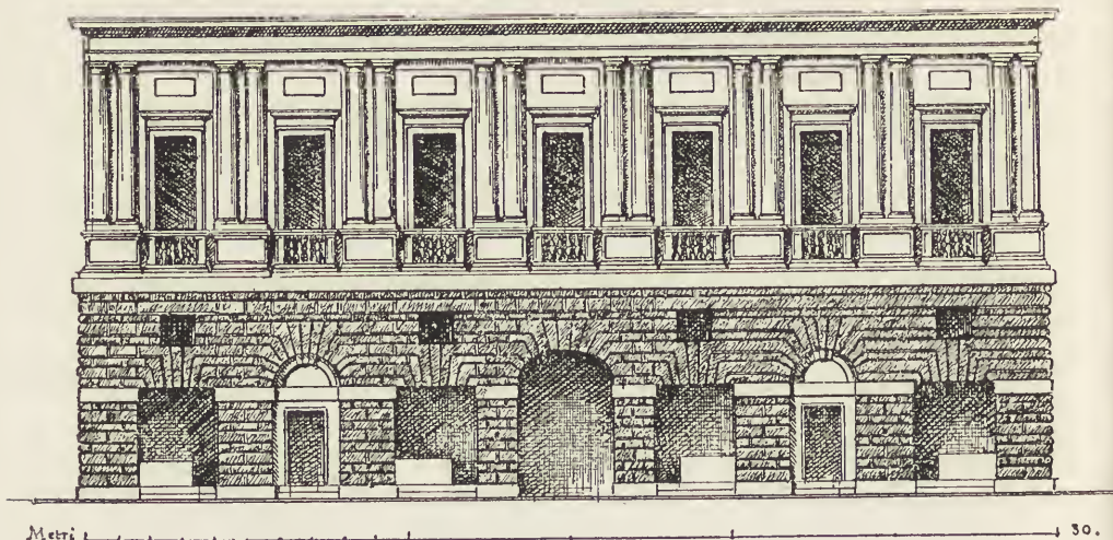
Fig. 189. Pal. Vidoni-Caffarelli in Rom. Nach Geymüller.
