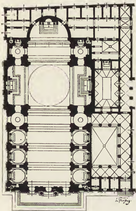
Fig. 137. Il Gesù in Rom. (Nach Gurlitt.)
