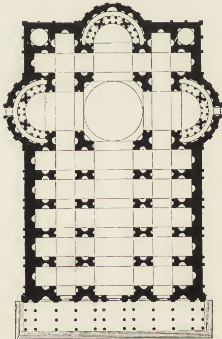
Fig. 94. St. Peter. Rafaels Grundriss. (Nach Serlios entstellter Reproduktion.)
