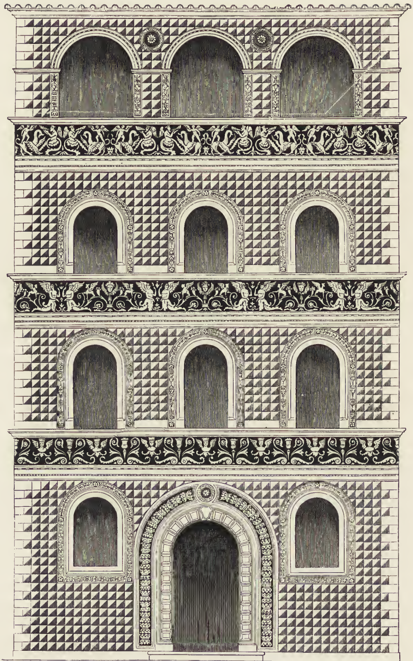
Fig. 237. Sgraffitofassade zu Florenz.
