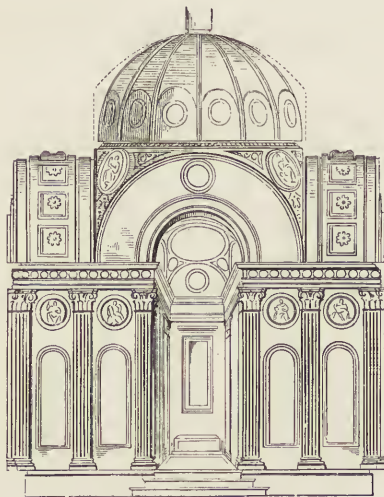
Fig. 76. Capp. Pazzi zu Florenz. Längsschnitt. (Nohl.)
