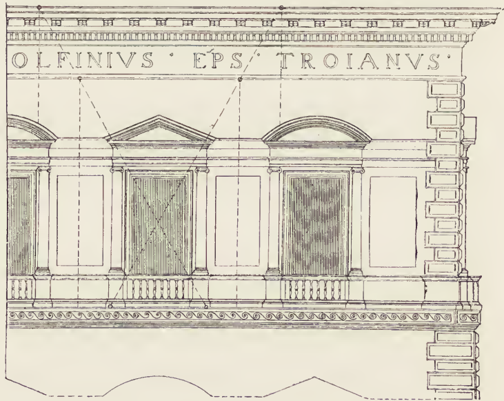
Fig. 61. Vom Pal. Pandolfini zu Florenz. (Nach A. Thiersch im Handb. der Archit.)
