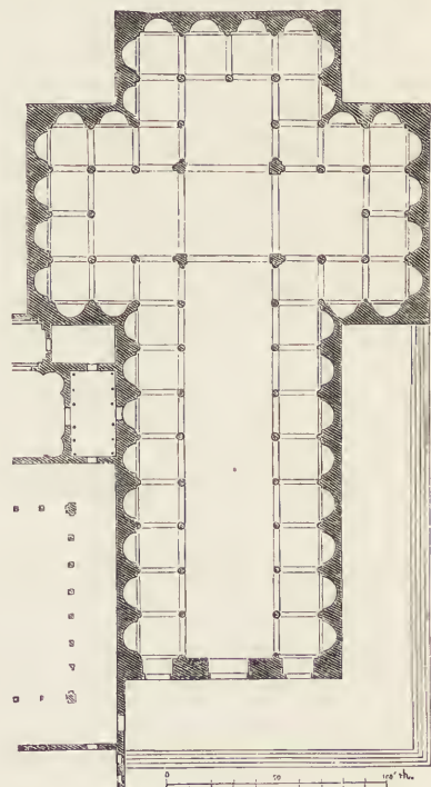
Fig. 123. S. Spirito zu Florenz. Grundriss.
