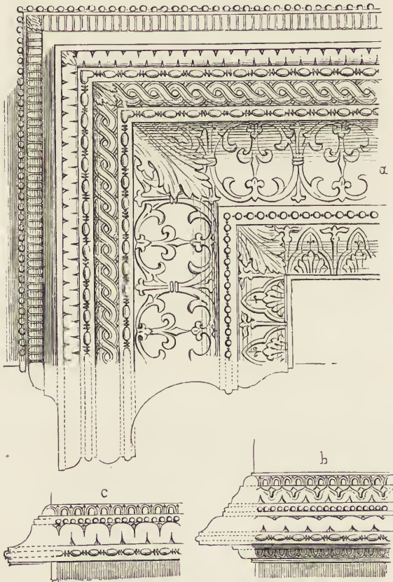
Fig. 299. Kapelle der Cancelleria. Details. (Nohl.)
