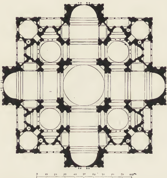
Fig. 92. St. Peter. Bramantes erster Grundriss.
