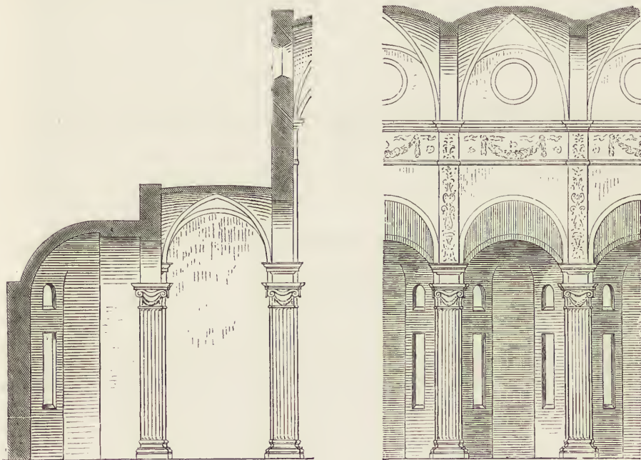
Fig. 143 und 144. S. Giovanni in Parma. Quer- und Längenschnitt. (L.)
