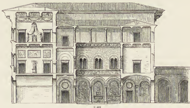
Fig. 172. Pal. Riccardi zu Florenz. Durchschnitt.
