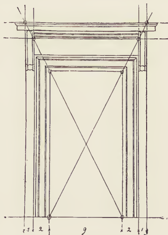
Fig. 62. Thürumrahmung. (Nach A. Thiersch.)
