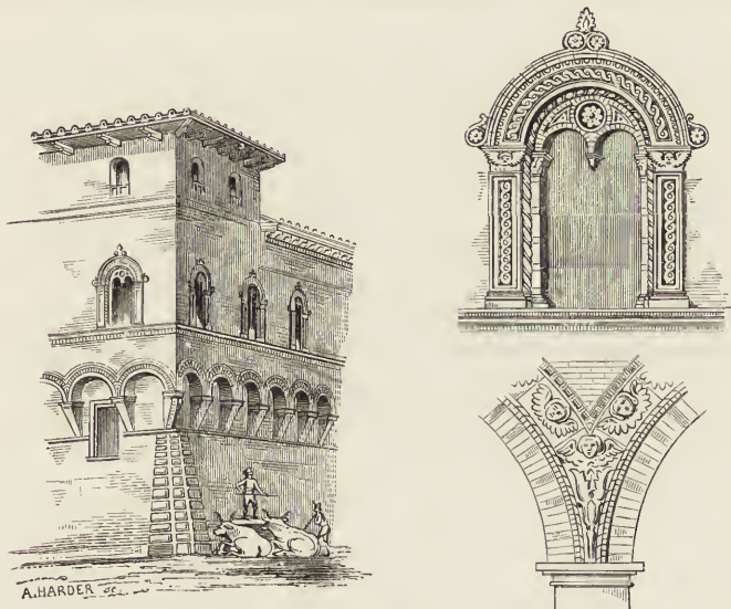
Fig. 33. Palast zu Bologna. (Nohl.)
