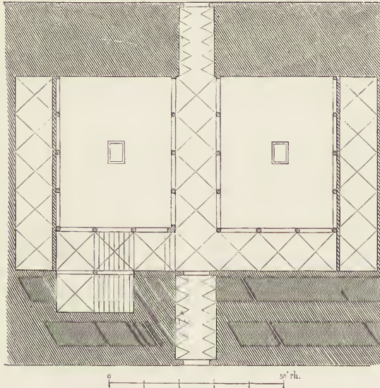
Fig. 179. Pal. Pizzardi zu Bologna. (L.)
