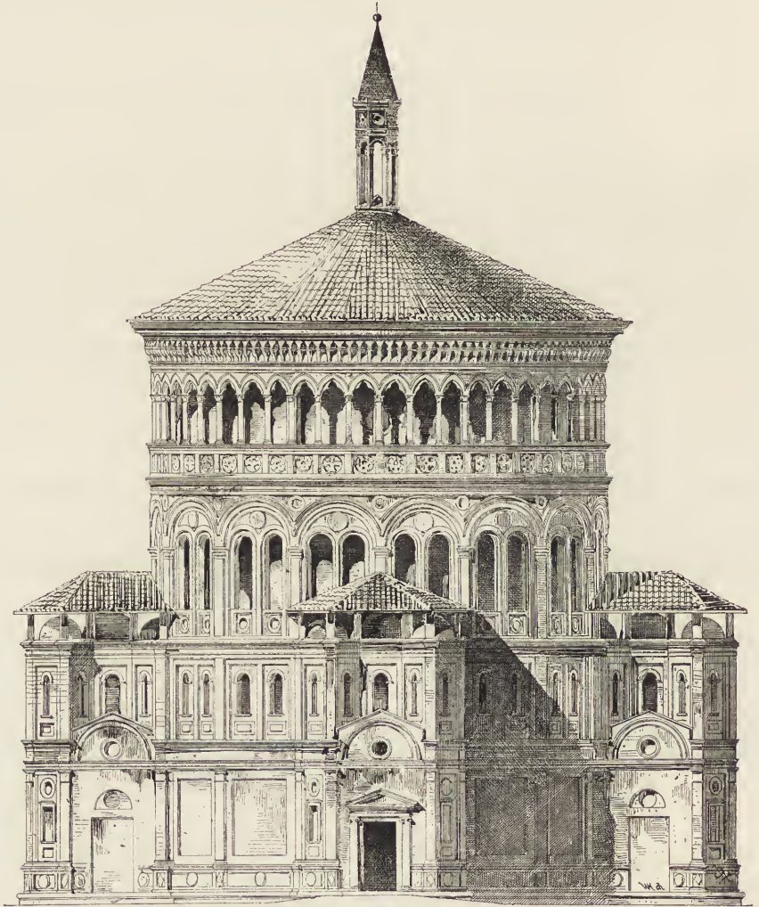
Fig. 39. Madonna della Croce bei Crema. (Nach Paravicini.)
