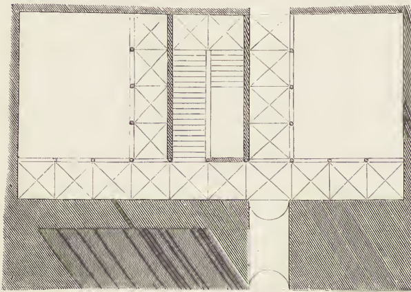
Fig. 180. Pal. Fantuzzi zu Bologna. (L.)
