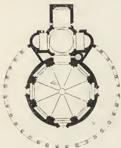
Fig. 102. Madonna di Campagna bei Verona. (L.)
