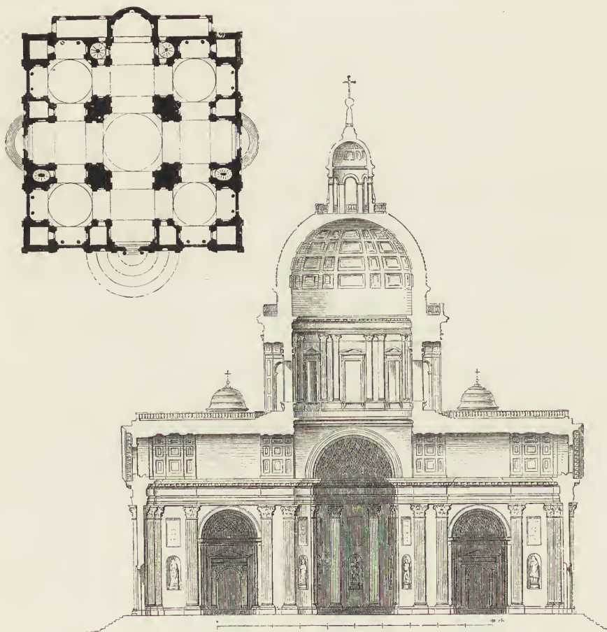
Fig. 107 und 108. Madonna di Carignano in Genua.
