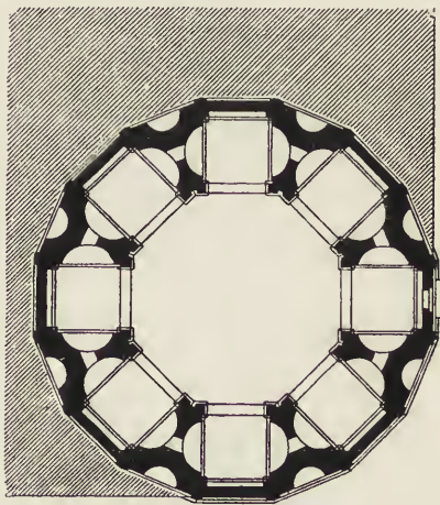
Fig. 78. S. Maria degli Angeli zu Florenz.
