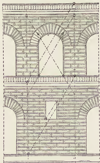
Fig. 65. Vom Pal. Pitti zu Florenz. (Nach A. Thiersch im Handb. d. Archit.)
