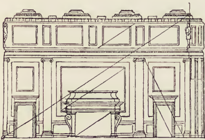
Fig. 71. Hauptsaal des Pal. Massimi in Rom. (Nach A. Thiersch im Handb. d. Archit.)
