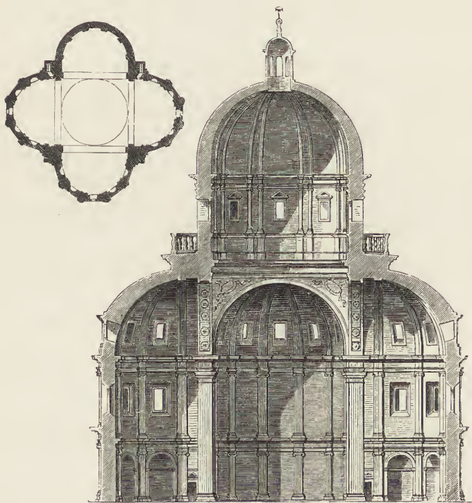
Fig. 97 und 98. Consolazione zu Todi.
