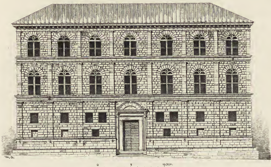
Fig. 23. Palazzo Piccolomini zu Pienza. (Nach Mayreder.)
