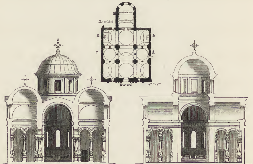
Fig. 86-88 S. Maria de' Miracoli zu Brescia. (Nach Herdtle.)
