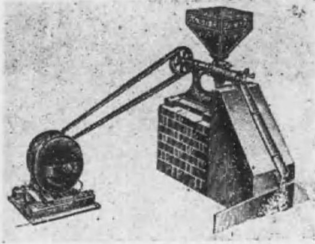
電動機裝置ノ圖
