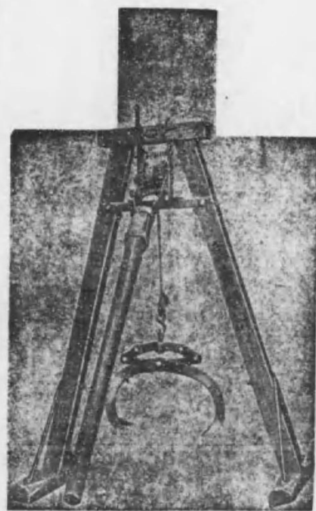
田中式株拔取機
