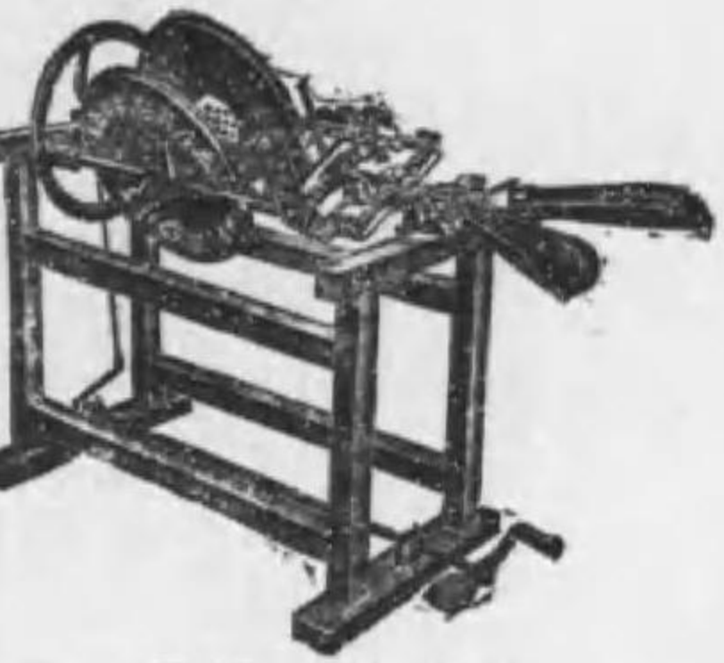
本庄式製繩機
