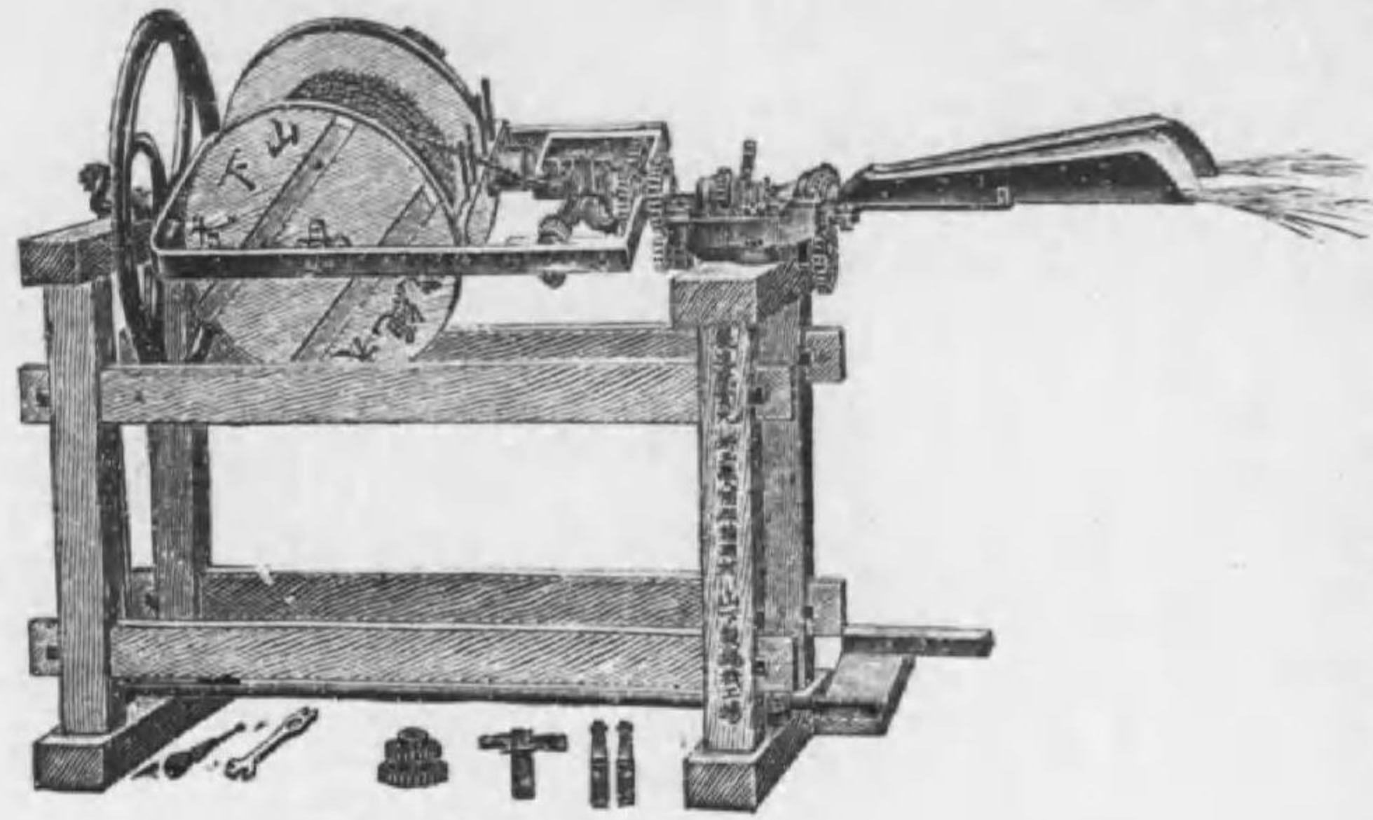
(圖之機繩製式下山)
