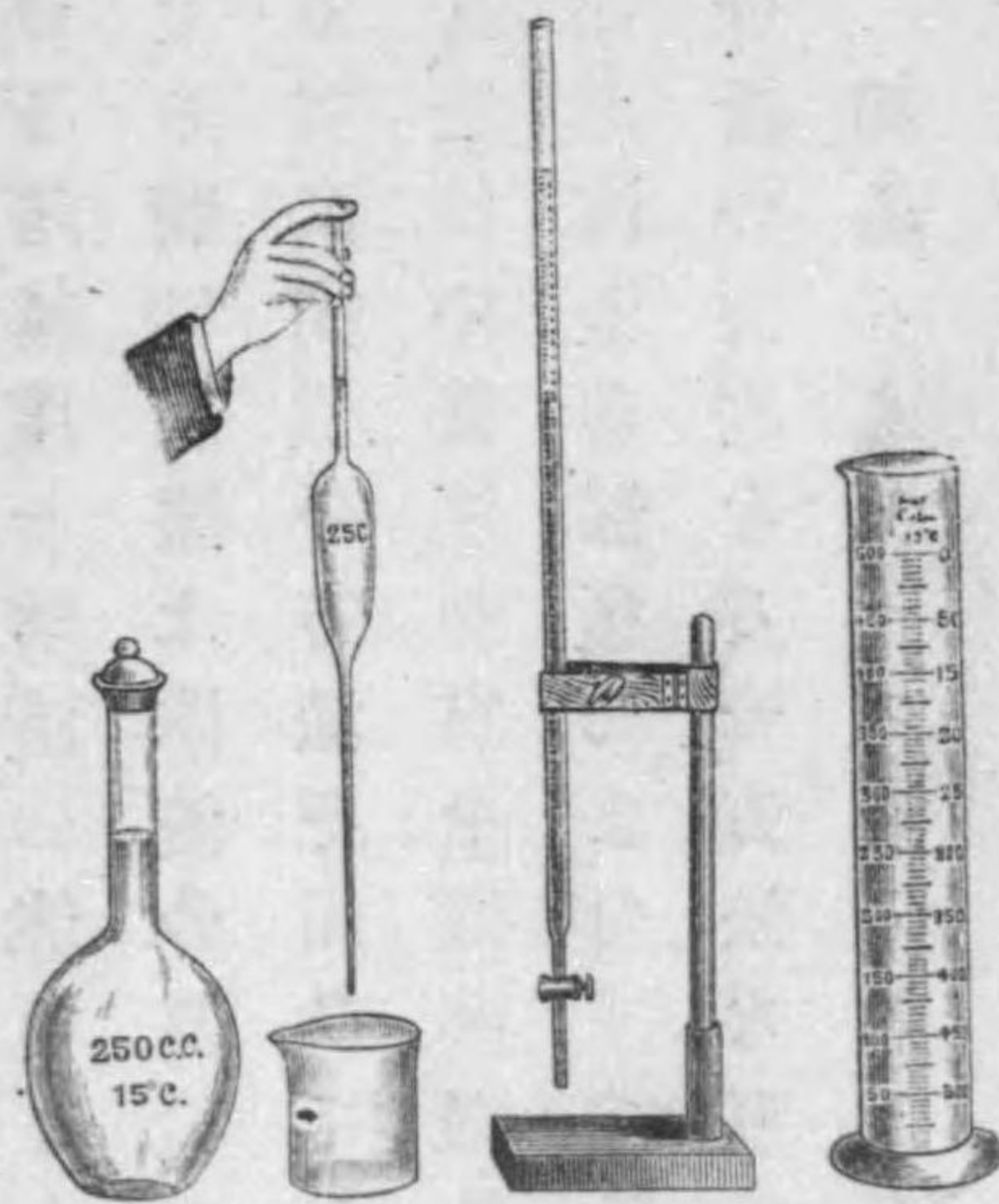
第四一圖 容量分析に用 ふる器具 劃度圓筒 ビュレット ピペット ピーカー 容量壺
