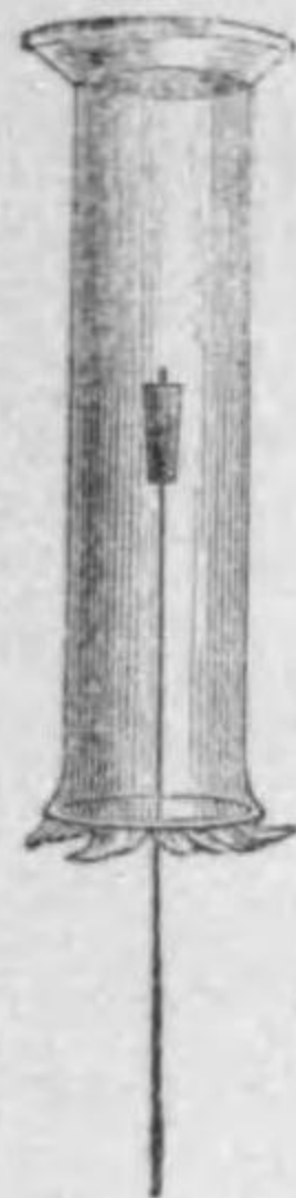
第一〇圖 水素中に燭火 を挿入す
