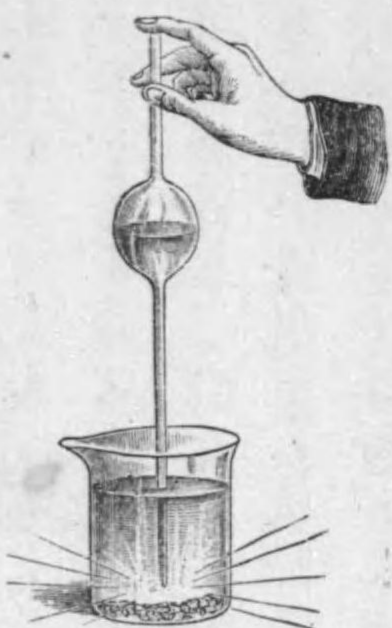
第六四圖 水中にて燐を 燃燒せしむ
