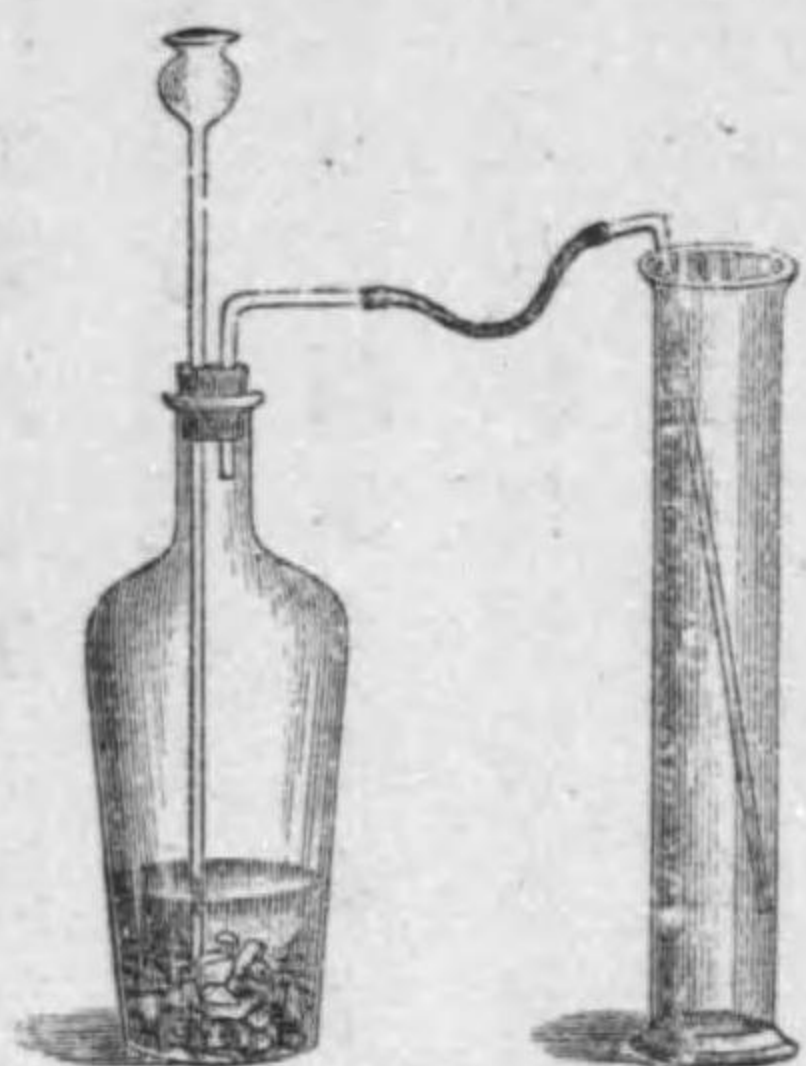
第二八圖 無水炭酸の製法
