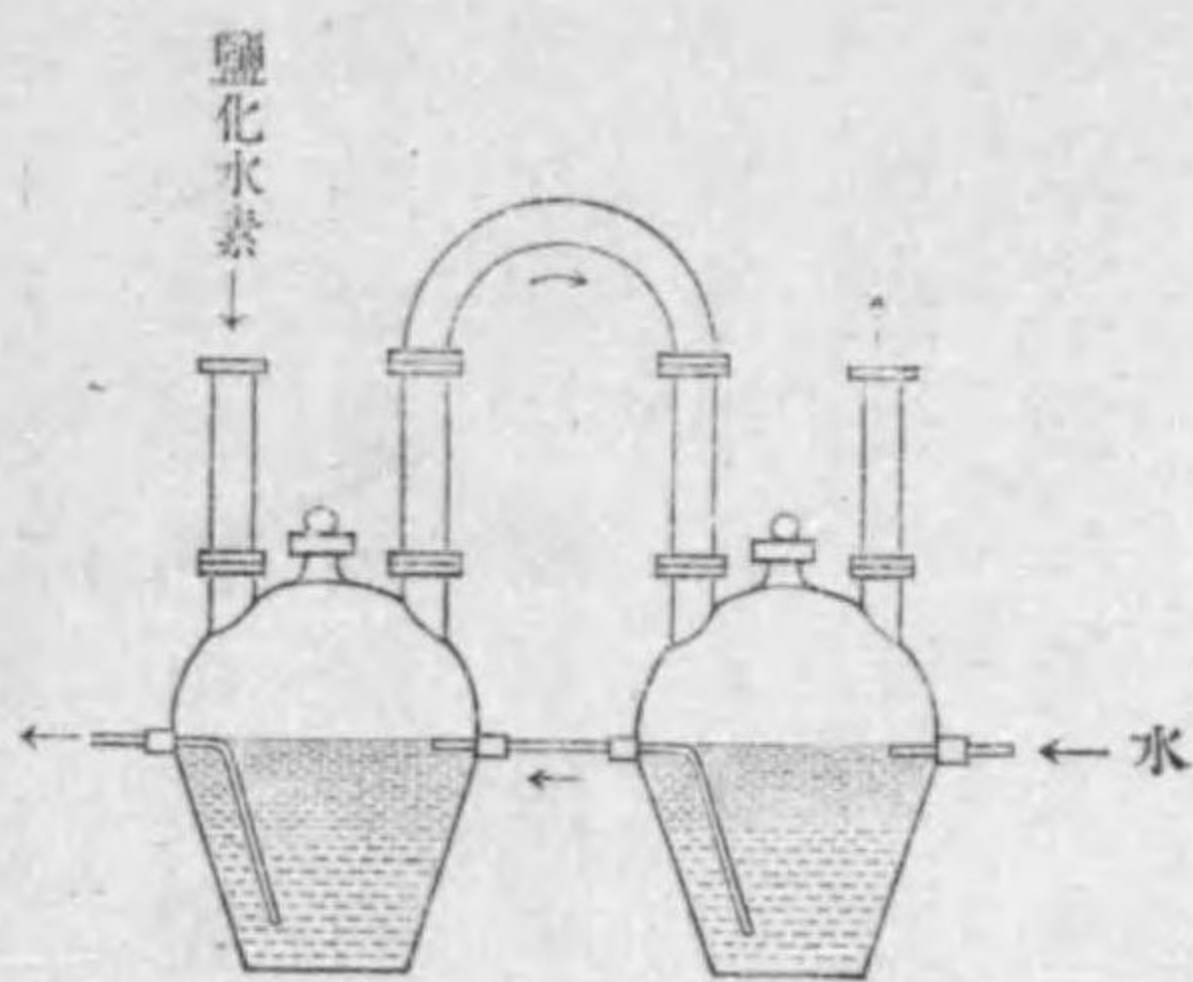
第三六圖 鹽化水素吸收裝置
