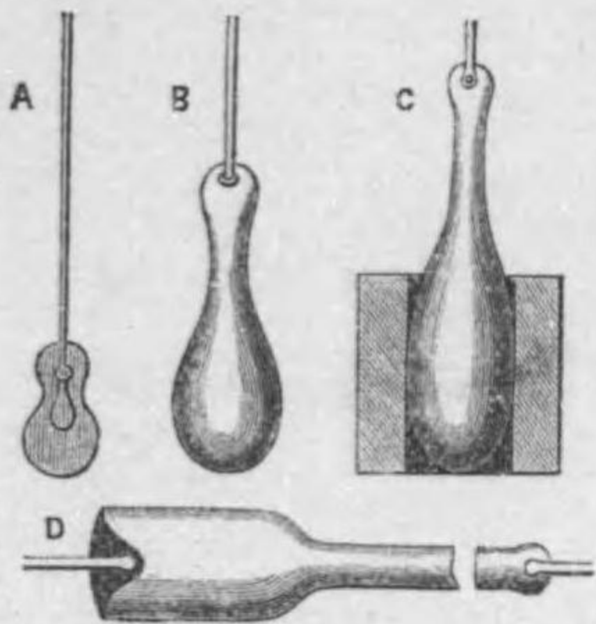
第五七圖 硝子壘製造順序
