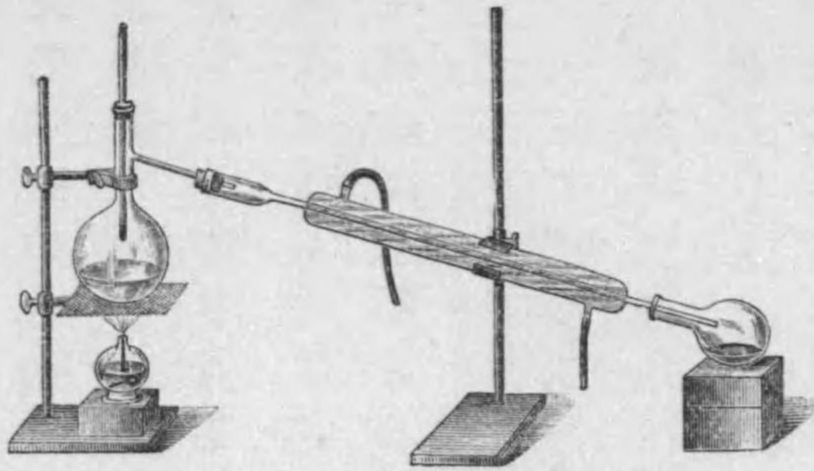
第一四圖 實驗場に於ける蒸溜装置
