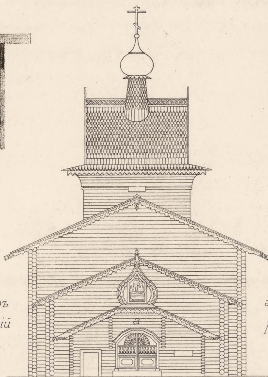
ЗАПАДНЫЙ ФАСАДЪ ЦЕРКВИ ВЪ С. ЧЕРЕВКОВѢ FAÇADE OCCIDENTALE DE L'ÉGL. À TSCHERÉWKOWO
