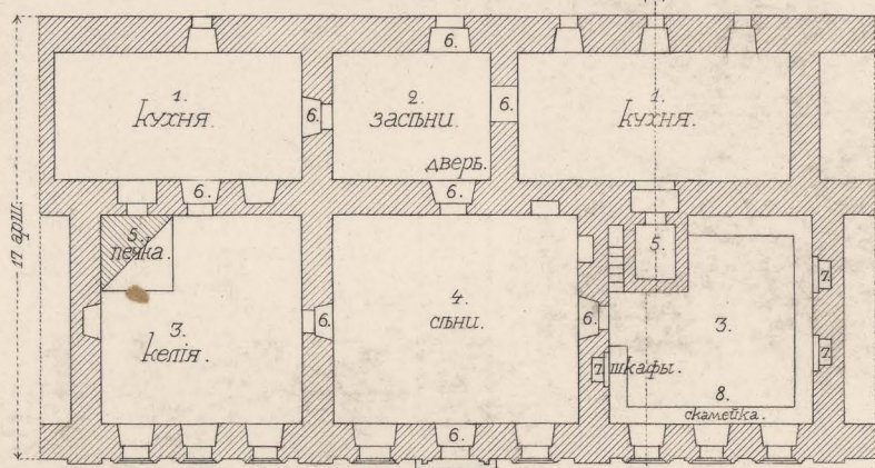
GALERIE DES DÉPÔTS DU MONASTÈRE SPASSO-PRILUTZKOÏ À WOLOGDA.
