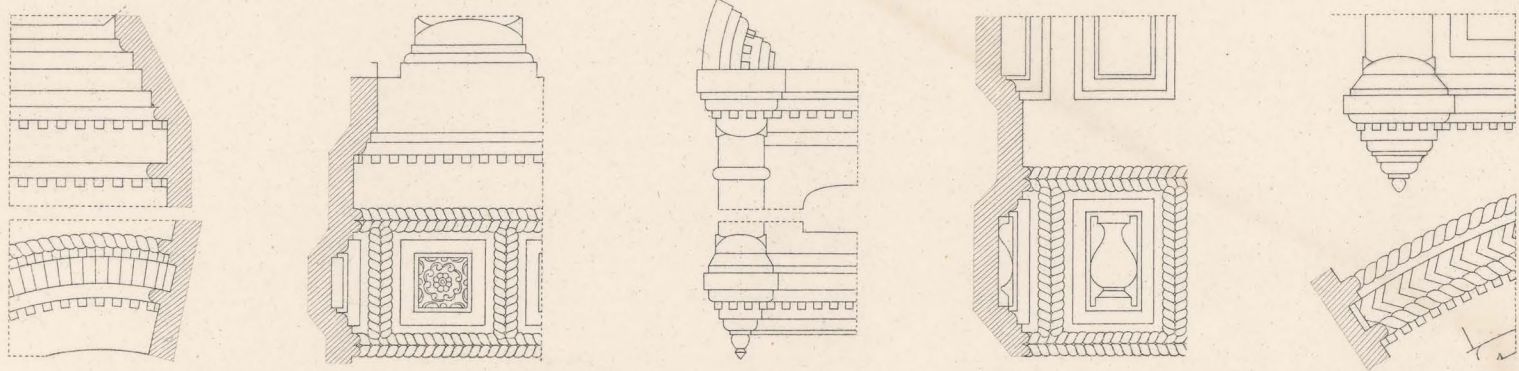
ДЕТАЛИ Ц. ВОСКРЕСЕНІЯ ХРИСТОВА въ г. Ростовъ Ярославской гув.
