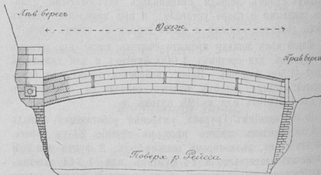
Фиг. 2. Крѣпостной мостъ сѣвернѣ «Урнерлохъ» (видъ съ южной стороны).
