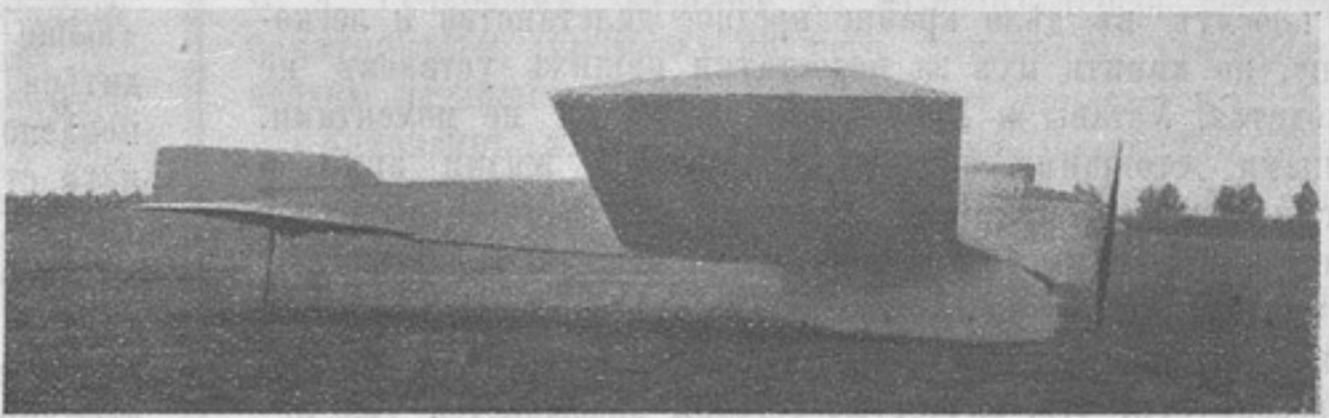
Новый монопланъ Латама. Видъ спереди, сзади и сбоку. Весь построенъ безъ металлическихъ растяжекъ. Размѣры громадные: 22 арш. въ ширину и 16 въ длину; ширина крыльевъ у основанія 5,5 арш. и по концамъ—4,5.
