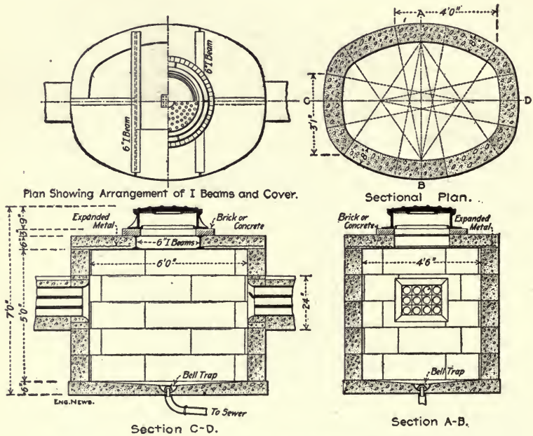
Fig. 267.—Concrete Block Manhole.
