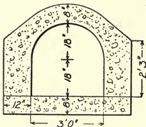
Fig. 171.—Small Culverts, Pennsylvania R. R.
