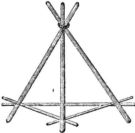
Рис. 9. Пирамида для сушки сѣна.
