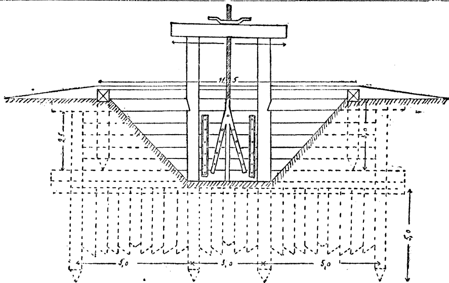
Рис. 5а. Простой шлюз главной канавы.
