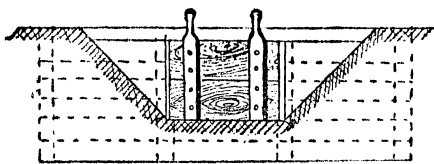
Рис. 5б. Простой шлюз въ осушит. канавѣ (боковой).
