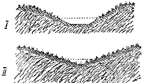
Рис. 4. Правильная форма канавы (с более отлогими стбнками).
