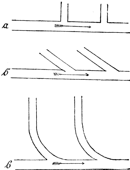
Рис. 6. Соединеніе боковыхъ канавъ съ главной: а—неправильное, б и в—правильное.
