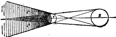
Полное Л. з. S—солнце, E—земля, M—луна, P—полутѣнь.
