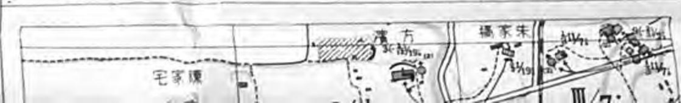
圖要戰隊大一第隊聯九十第兵步
