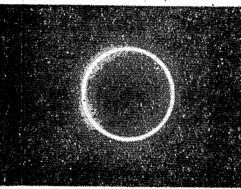
这是四月二十九日在喀喇昆仑山海拔五千二百米的观测点上拍摄的日环食照片。新华社记者摄。
