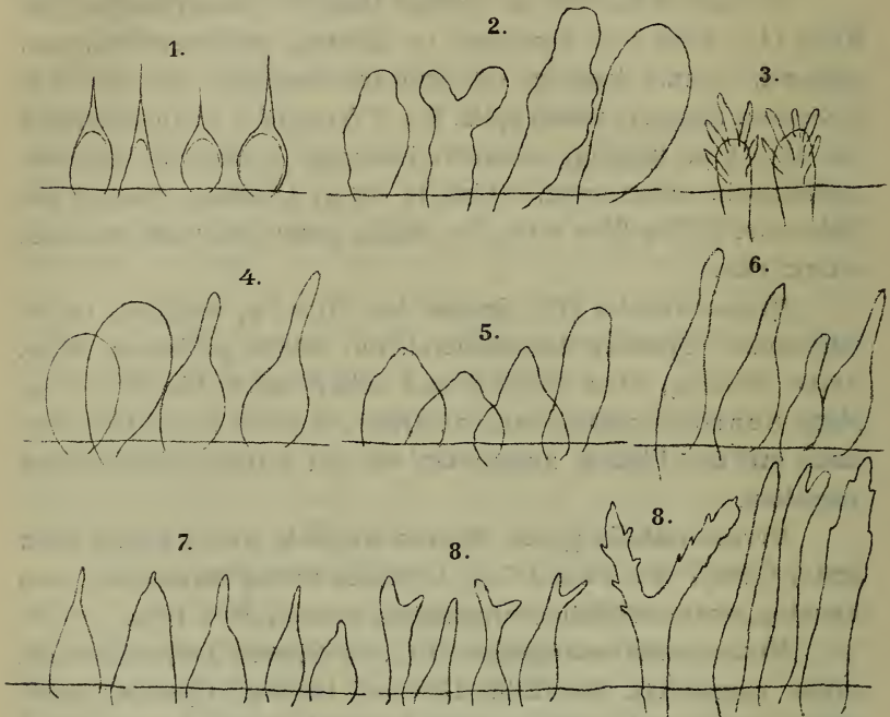
Fig. 3. Mycena -Cystiden.
