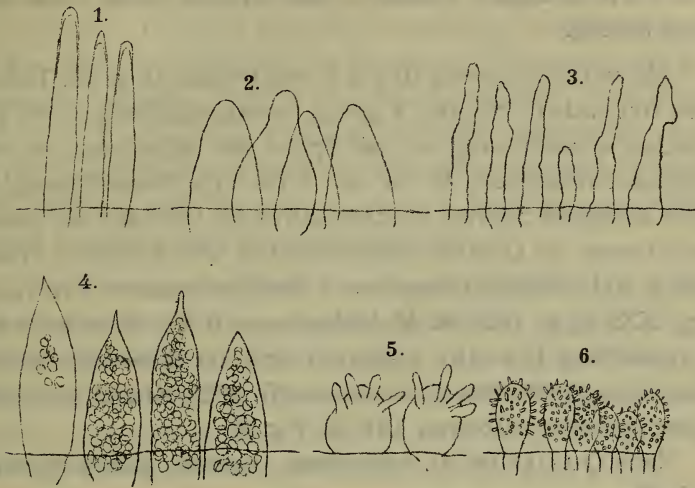
Fig. 2. Mycena -Cystiden.
