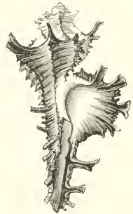
Fig. 11. — Rocher scorpion.
