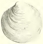
Fig. 7 - Félanie rose
