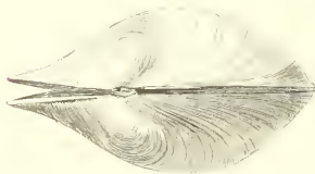
Fig. 7 — Maetra élégante
