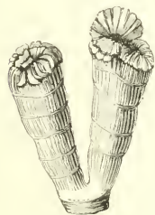
Fig. 291. — Caryophyllie.
