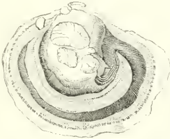
Fig. 201. — Anomie Ehippium.
