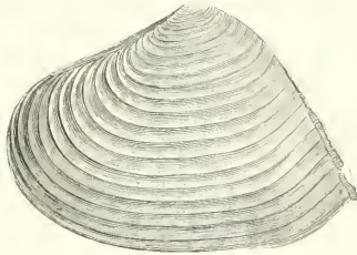
Fig. 2 — Mactre striée.
