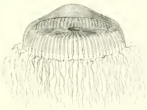
Fig. 284. — Ecuorée bleue.
