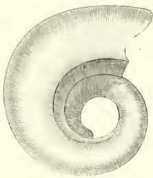
Fig. 67. — Nautilite subsilloné.
