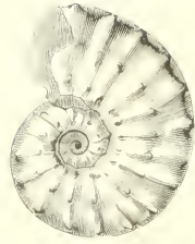
Fig. 5 -- Ammonite variante.
