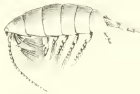
Fig. 54. — Pontie atlantique.
