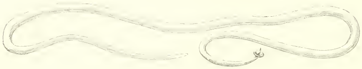
Fig. 296. — Strongle géant.
