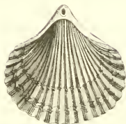
Fig. 6 — Rhynchonelle déprimée
