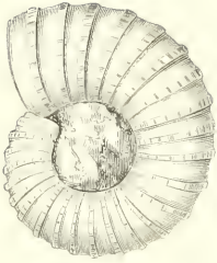
Fig. 1 — Ammonite mamillare.
