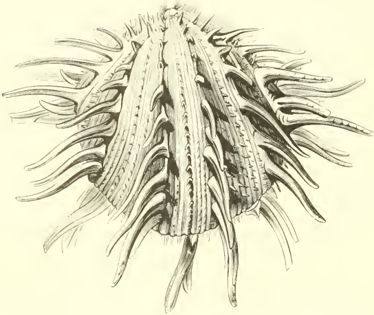
Fig. 2. — Spondyle royal
