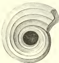
Fig. 89. — Nautilé multicaréné.
