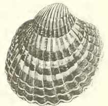
Fig. 12. — Bucardé no-rouse .
