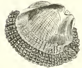
Fig. 9 — Myocame anomioide
