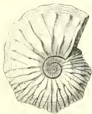
Fig. 66. — Ammonite pustuleuse.
