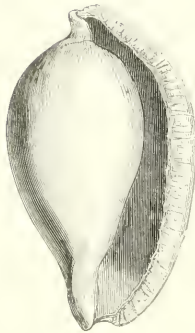
Fig. 5. — Ovale aul.
