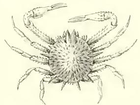
Fig. 1. — Arémie hérisson.
