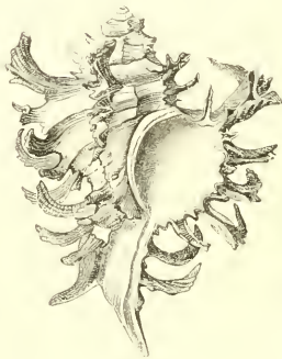
Fig. 148. — Rocher enlève
