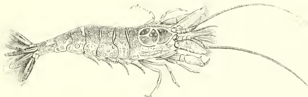
Fig. 14. -- Crustacé commun.
