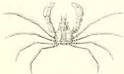
Fig. 4C. -- Inaque dorynque.
