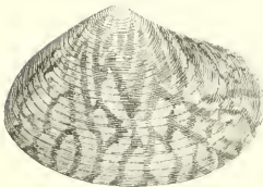
Fig. 10. — Fonace ni-roe .
