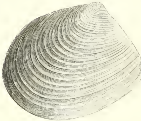
Fig. 7 — Mactre élégante
