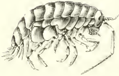
Fig. 4. — Talctre sauteur
