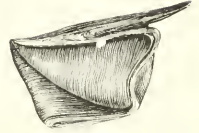
Fig. 6 — Bradiolites fissirostre
