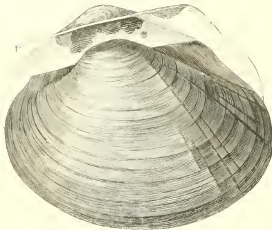
Fig. 2 — Amudonte glauque
