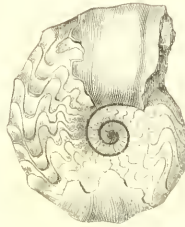
Fig. 105. — Goniatite noueuse.
