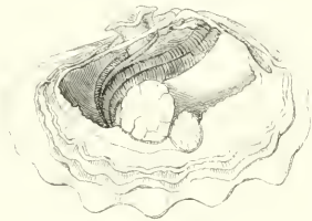
Fig. 202. — Tridacne Safran.
