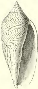
Fig. 9. — Volute zébrée
