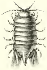
Fig. 1 — Cymodocé armé.
