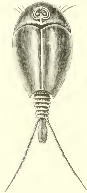
Fig. 3 — Apus canaliculatus
