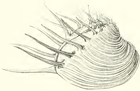
Fig 4 — Cythérée Dione.
