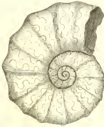
Fig. 104. — Goniatite noueuse.
