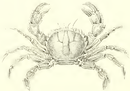
Fig. 48 — Portune étrille.
