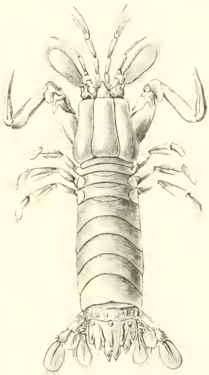
Fig. 2 — Gonolactyle stylifère
