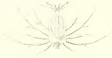
Fig. 1 — Phyllosome commun
