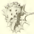
Fig. 8 — Bicnule trachioïde
