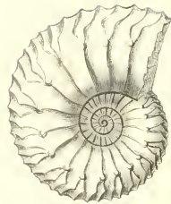
Fig. 5 — Ammonite cordiforme.
