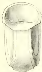
Fig. 88. — Nautilé multicaréné.
