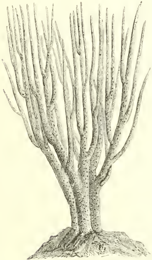
Fig. 289. — Lithophyton américain.
