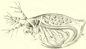
Fig. 4 — Daphnie puce
