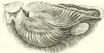
Fig. 207. — Gryphole arqué
