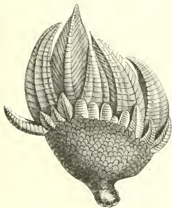
Fig. 43. — Capitulum mitella.
