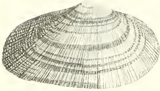
Fig. 1 - Sangumolaire rugueuse
