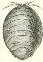
Fig. 2 — Cassidine type
