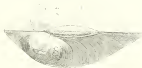
Fig. 225. — Cyrène verte .
