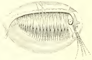
Fig. 5 — Limnische d'Hermann.
