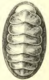
Fig. 146. — Osecabtron géant.
