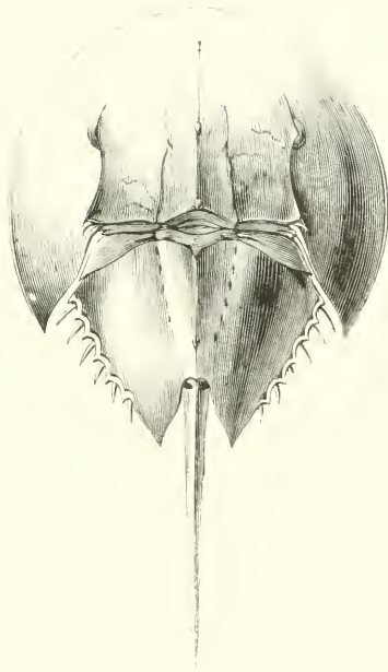
Fig. 1 — Limule polyphème
