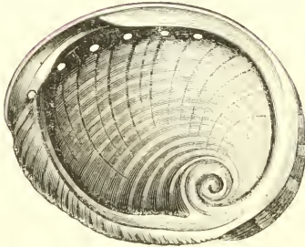
Fig. 145. — Haliotide excavée.
