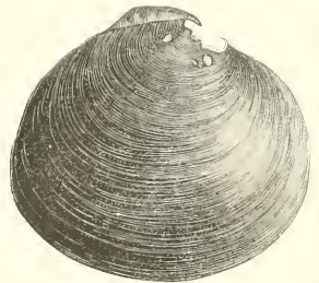
Fig. 11 — Cyrène verte.
