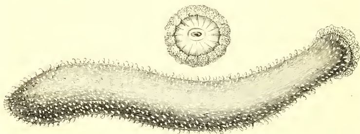
Fig. 274 — Holothurie tuberculeuse.
