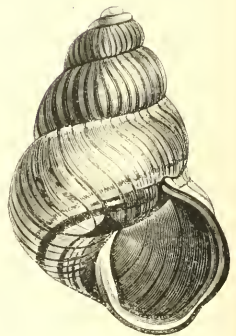
Fig. 149. — Baline daplus
