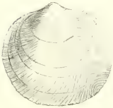
Fig. 6 — Lucine bivarripiée
