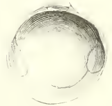
Fig. 9 - Félanie rose
