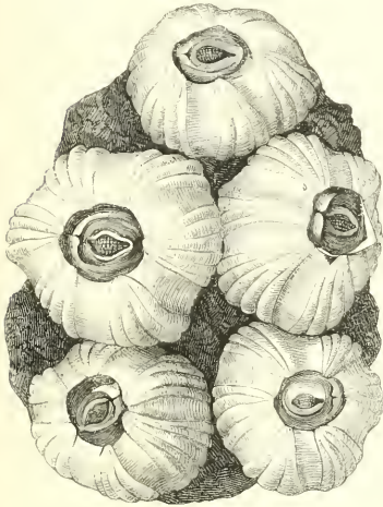
Fig. 48. — Coronule Diadème.
