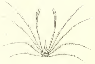
Fig. 5. — Leptopode sagittaire
