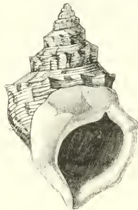
FIG. 196. — Struthiolaire nodulense.
