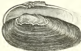
Fig. 8 — Glauconome tridenté
