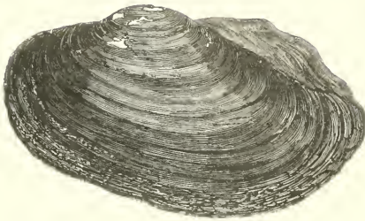
Fig. 4 Trochantele auréole
