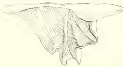
Fig. 4 — Bradiolites fissirostre
