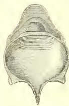
Fig. 59. — Hyalée tridentatée
