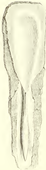
Fig. 4 — Bélemnite semi-rayée.
