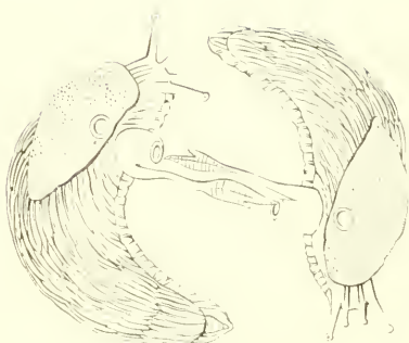
Fig. 4 — Limace rouge
