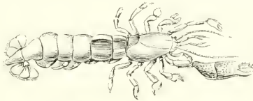
Fig. 24 — Callinasse souterraine.
