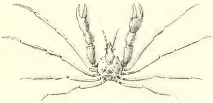
Fig. 2. — Stenorhynque lacheur .
