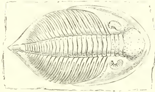
Fig. 52. — Asaphé caudigère-tuberculeuse.
