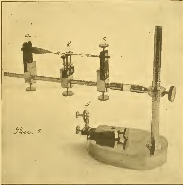
Рис. 1. Міоскопъ.
