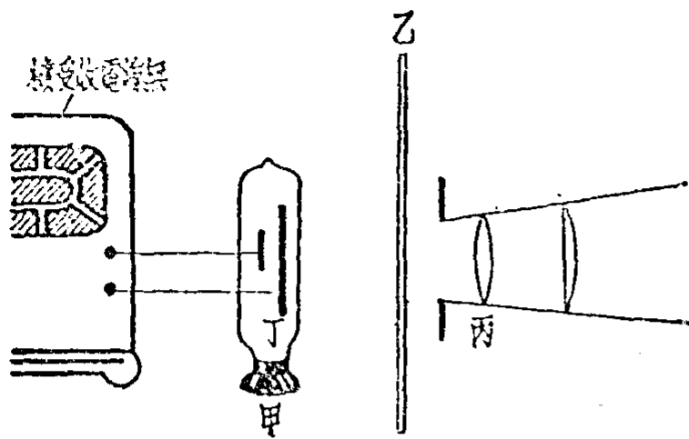
電 視 接 收 的 原 理 (圖一十)
