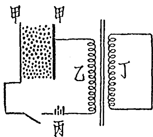
機音微 (二十圖)
