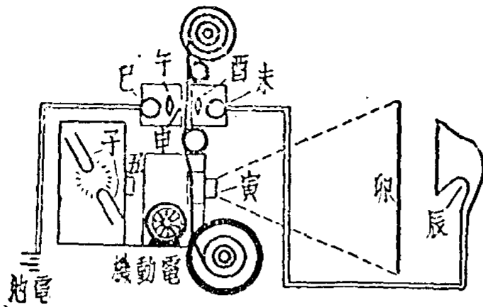
機映放影電聲有 (五圖)
