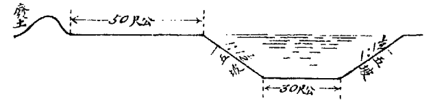
第二引河橫剖面標準圖
