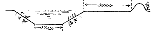
第一引河橫剖面標準圖
