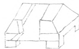
齊心料 泥道拱 上用
