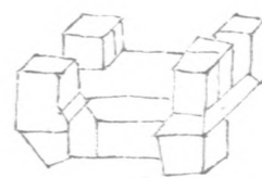
齊心料 令拱 上用
