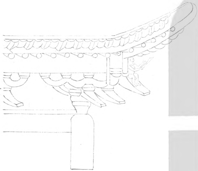
鋪作轉角正樣第九 殿閣亭榭等轉角正樣四 鋪作壁內重拱插下昂
