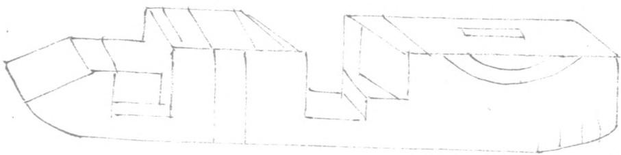
慢拱與華頭子相列 外跳用七鋪作 以上隨跳加長
