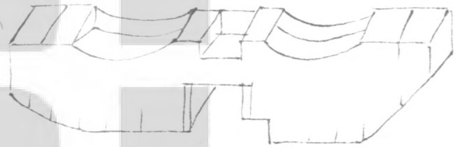
瓜子拱 用 外跳
