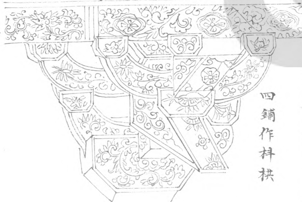
五鋪作拱
