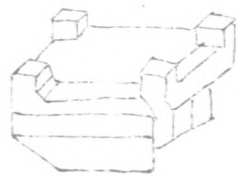
齊心料 泥道拱 上用
