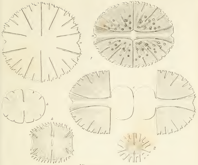
Micrasterias
