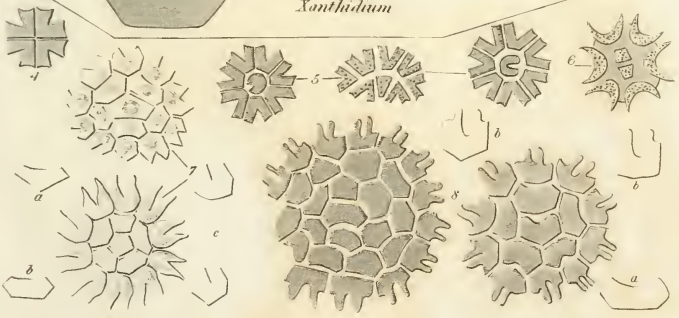
Radiastrum.
