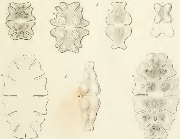
Euastrum
