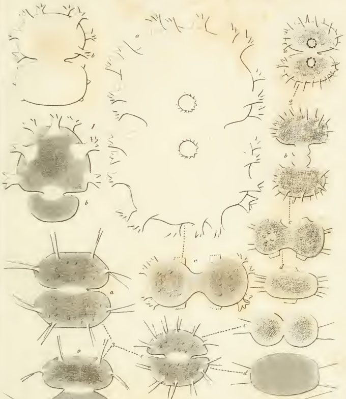
Xanthidium
