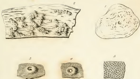
Rhododermis Drummondii
