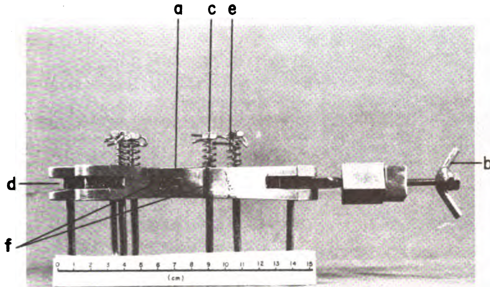
Figure 2. Déclencheur à 4 pistons égaux: déclenchement à une profondeur. (a) pivot latéral, (b) verrou, (c) piston, (d) alvéole, (e) ressort, (f) orifice central.
