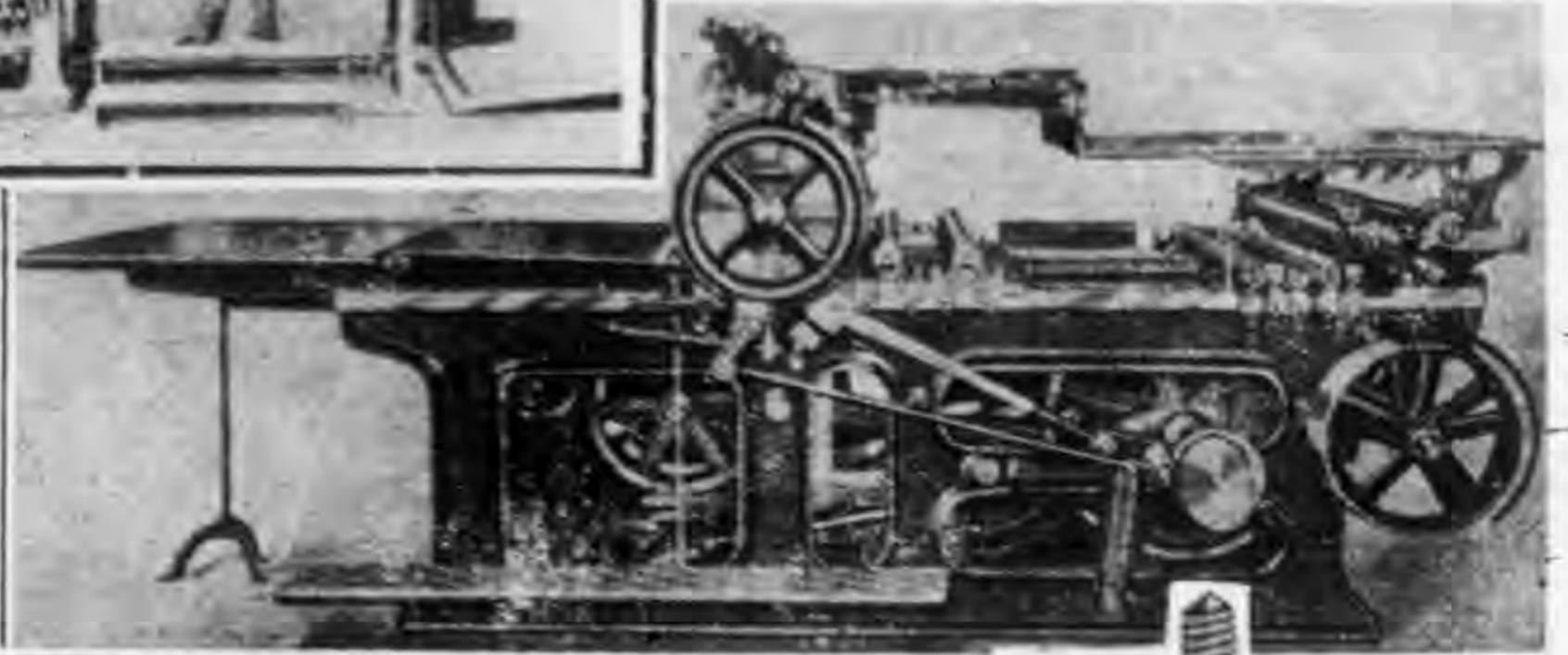
↑ 一八四六年美國李卓賀氏 最早發明之輪轉機
