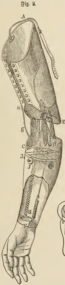
Fig. 2-4. Charrières künstlicher Vorderarm. Fig. 5 u. 6. Bly's künstliches Bein.
