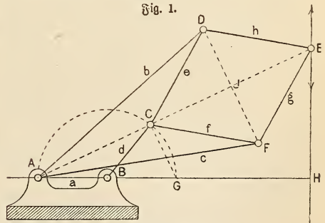
Geradsführung von Peaucellier.
