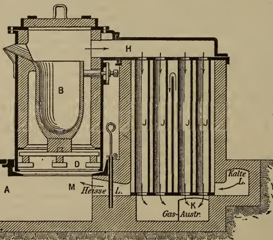
Tiegelofen
