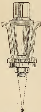
Gewöhnlicher Hahn.
