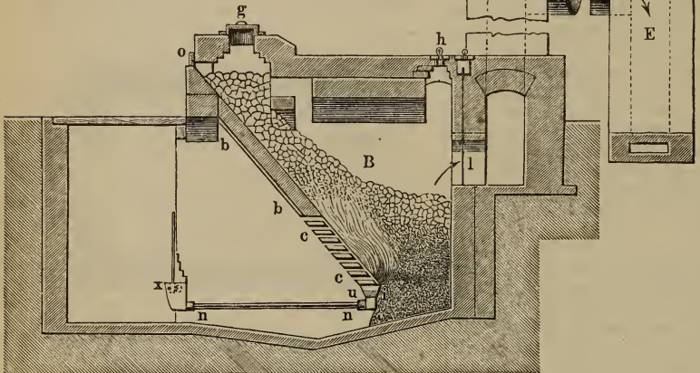
Siemens'scher Regenerativgasofen für Kohlen- und Torffeuerung.
