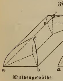
Muldengewölbe.
