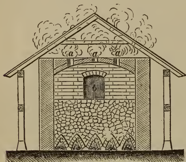
Gipsöfen
