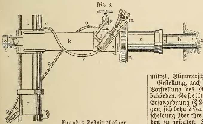
Brandt's Gesteinsbohrer.
