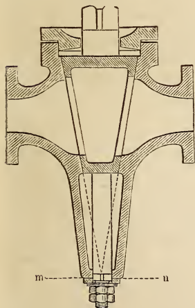
Collmanns Hahn.
