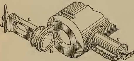
Kolbenverschuß.
