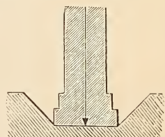
Fig. 17. Wagerechte Gründungsbasis.
