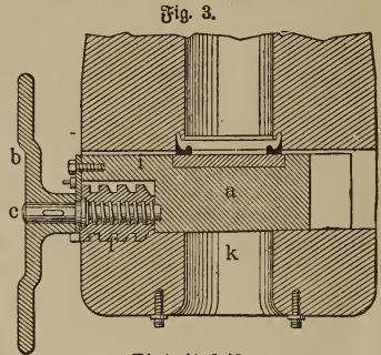
Fig. 3. Einheitskeil.
