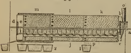
Marot'sches Sortiersieb. Durchschnitt.
