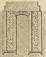
Fig. 14. Senkbrunnen in unfestem Baugrund.
