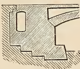
Fig. 22. Gezähnte, und Fig. 23. Getreppte Gründungsbasis von Widerlagspfählern.
