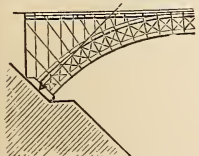
Fig. 18. Vorwärts geneigte, zur Druckrichtung normale Gründungsbasis.
