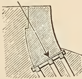
Fig. 18. Vorwärts geneigte, zur Druckrichtung normale Gründungsbasis.
