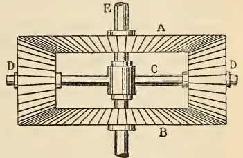
Regelräder-Umlaufgetriebe.
