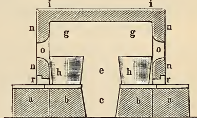
Fig. 1—3. Glasöfen für Holzfeuerung.
