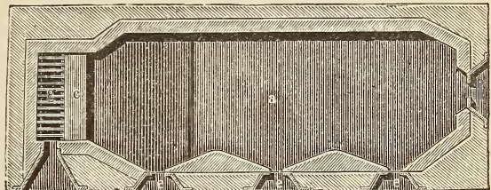
Rotierofen, Horizontaldurchschnitt.
