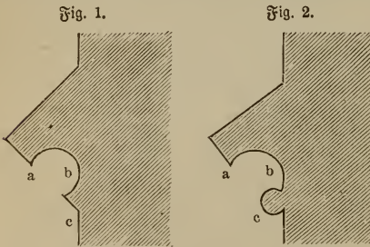
Hängende Gesimsplatten.
