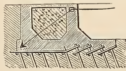
Fig. 24. Gebrochene, und Fig. 25. Gezähnte Gründungsbasis von Ankerpfählern.
