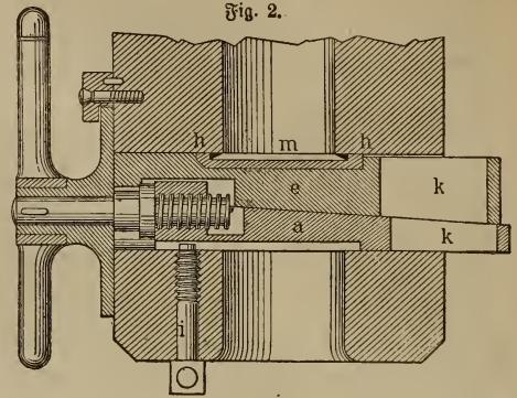
Fig. 2. Doppelkeilverschuß.
