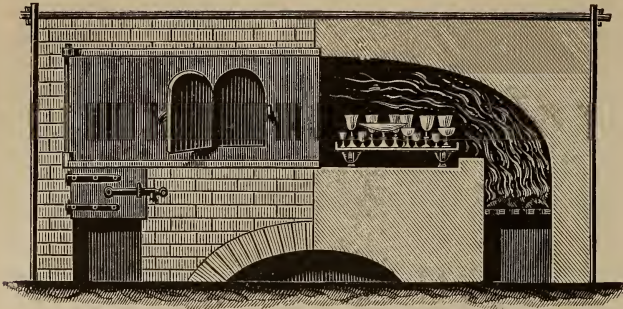
Fig. 17. Kühllofen für Bleiglas.
