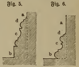
Fußgesimse.
