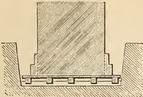
Fig. 2. Liegender Rost.
