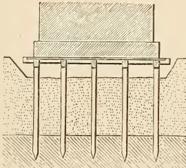
Fig. 9. Pfahlrost auf festem Untergrund.
