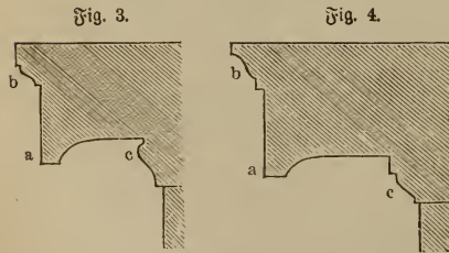
Liegende Gesimsplatten.
