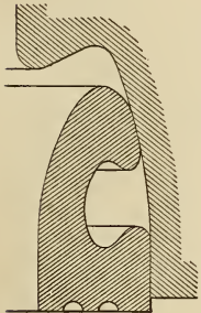
Liderungsring c/1873.
