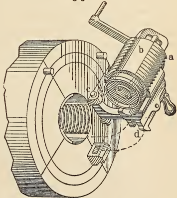
Schraubenverschluß
