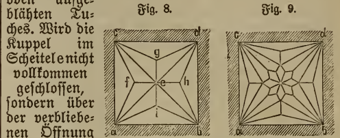
Sterngewölbe.
