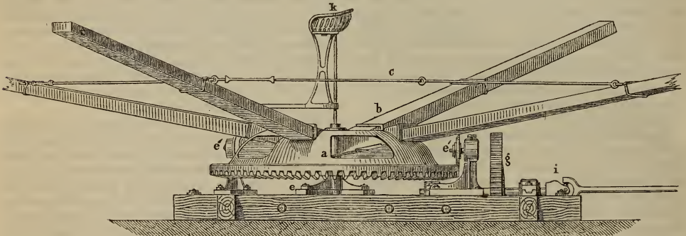
Pferdegöpel von Eckert, Seitenansicht.
