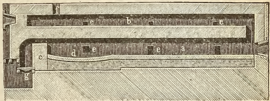
Röstofen, Rängendurchschnitt.
