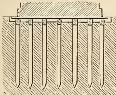
Fig. 15. Pfahlrost in unfestem Baugrund.
