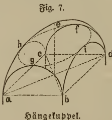
Hängekuppel.
