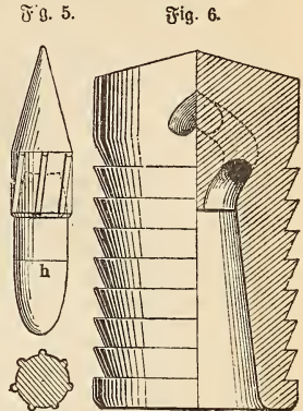
Fig. 5. Reichenbachs Langgeſchoß. Fig. 6. Turbinengeſchoß.
