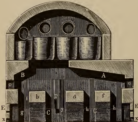
Fig. 5. Deutscher Glasofen, Durchschnitt.
