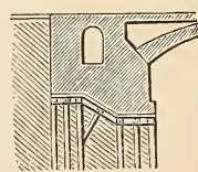
Fig. 21. Gebrochene Gründungsbasis.
