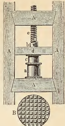
Fig. 13. Silberpresse zu Oker.
