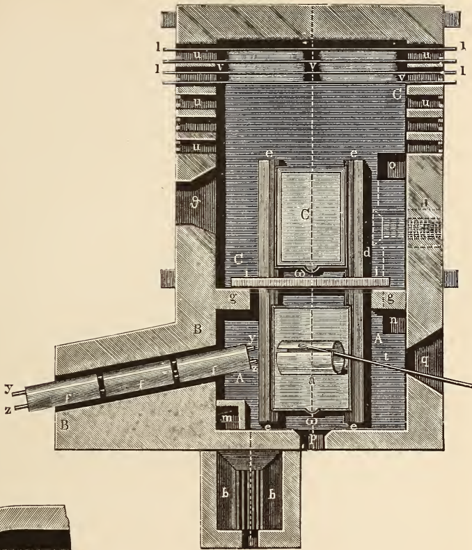
Fig. 20. Streckofen für Tafelglas, wagerechter Durchschnitt.
