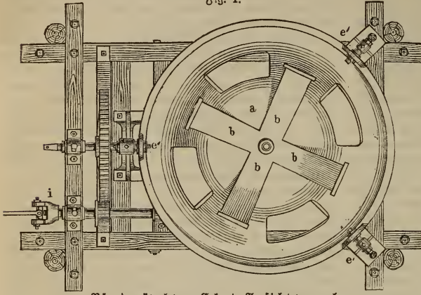
Pferdegöpel von Eckert, Ansicht von oben.
