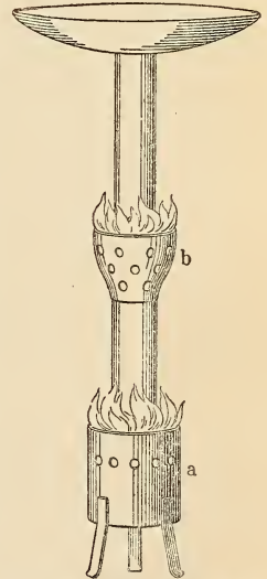
Müllers Apparat zur Erklärung der Geiserbildung nach Bunsen.
