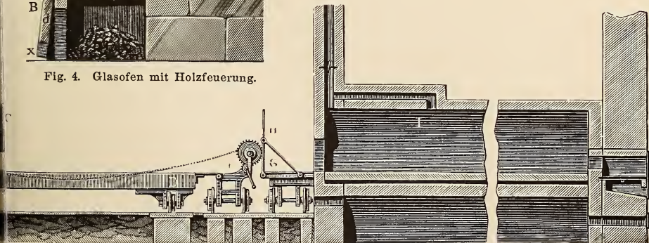
Fig. 22. Gießen des Spiegelglases.
