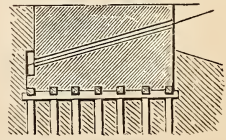
Fig. 24. Gebrochene, und Fig. 25. Gezähnte Gründungsbasis von Ankerpfählern.
