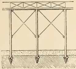
Fig. 6. Eiserne Schraubensäulen.
