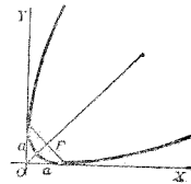
拋物線 PARABOLA
