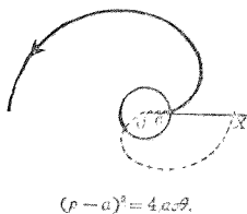
拋物線螺線 PARABOLIC SPIRAL
