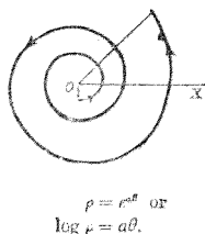
對數或等角螺線 LOGARITHMIC OR EQUIANGULAR SPIRAL
