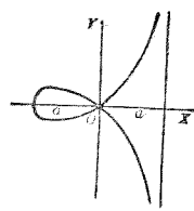
環索線 STROPHOID
