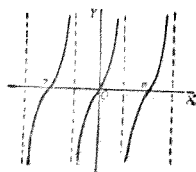
正切曲線 TANGENT CURVE
