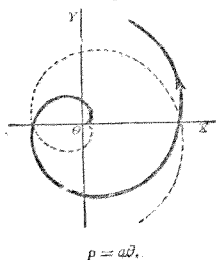
阿基米得之螺線 SPIRAL OF ARCHIMEDES
