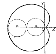
心臟線 CARDIOID
