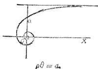
雙曲線或倒數螺線 HYPERBOLIC OR RECIPROCAL SPIRAL
