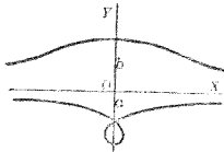
尼科美德之蚌線 THE CONCHOID OF NICOMEDES
