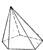
斜角錐
