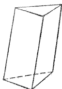
斜角柱
