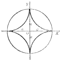
四支點之內切輪線 HYPOCYCLOID OF FOUR CURVES
