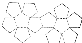
正十二面體
