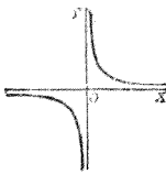
等邊雙曲線 EQUILATERAL HYPERBOLA
