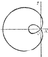
蠅線 LIMACON
