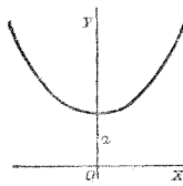
懸鏈線 CATENARY
