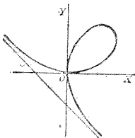
笛卡兒之蚌線 FOLIUM OF DESCARTES
