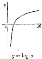
對數曲線 LOGARITHMIC CURVE
