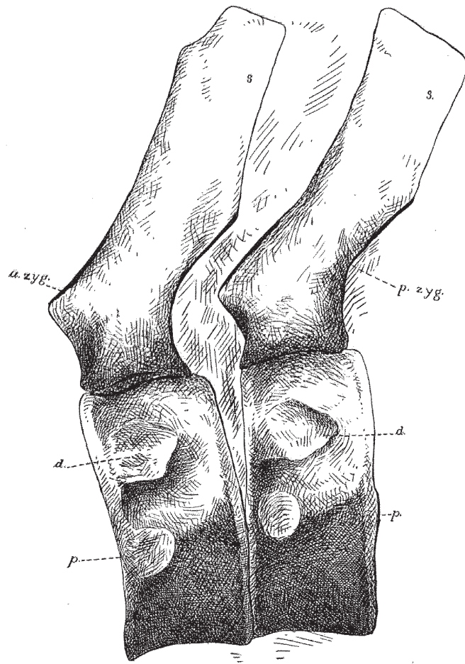
FIG. 13. Lateral view of anterior or median dorsals of Buptanodon robustus (No. 919). Type specimen. One half natural size. d. , diapophysis; p. , parapophysis; s. , spinous process; a.zyg. , anterior zygapophysis; p.zyg. , posterior zygapophysis.
