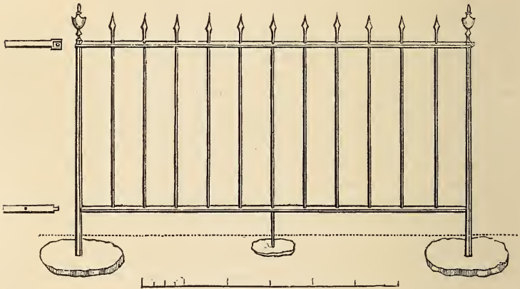
Fig. 333. Cast-iron Espalier-rail.
