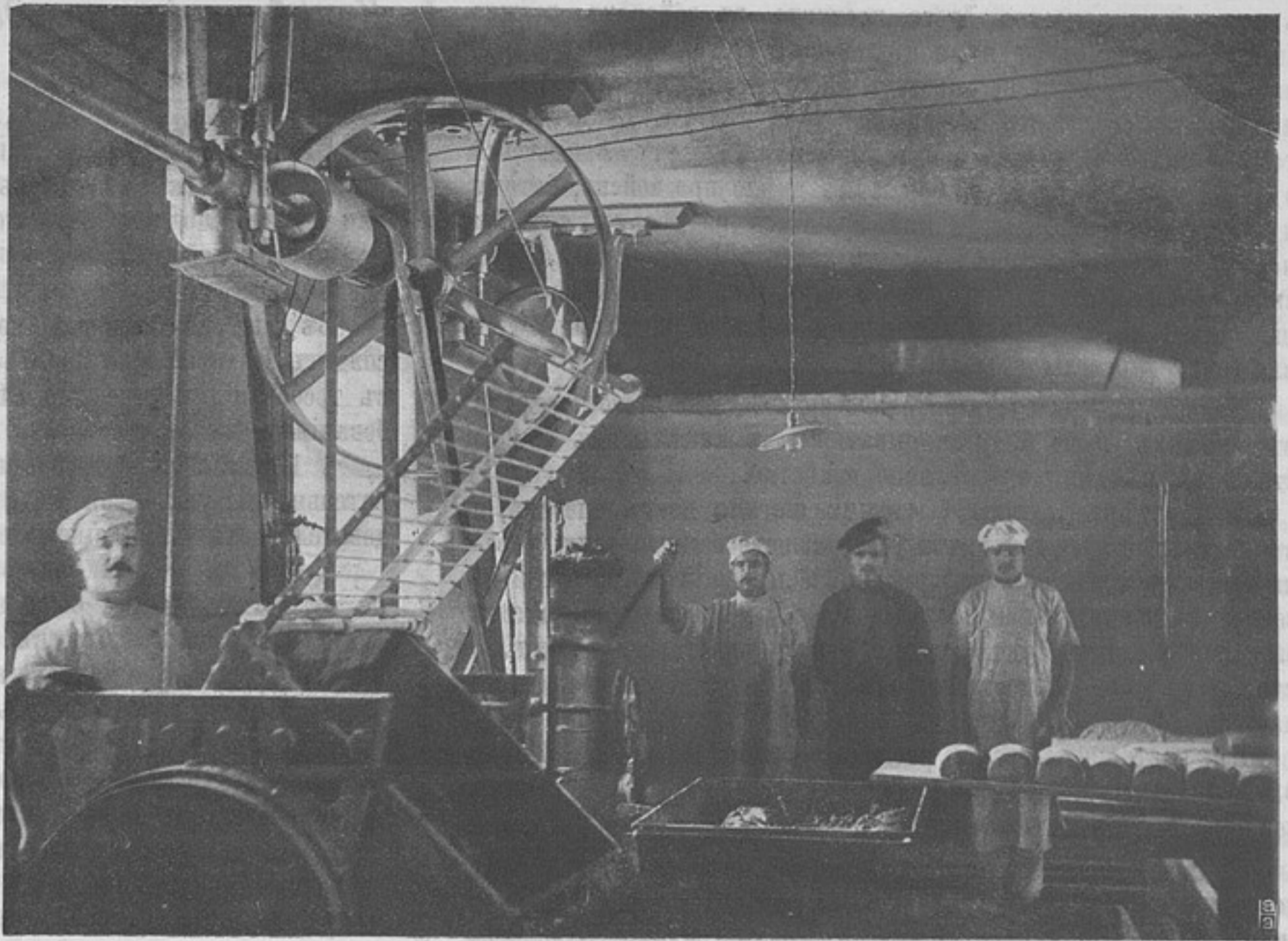
На лѣво тѣстомѣсилка, въ серединѣ моторъ и на право формовка. (Къ ст. «Солдатскій хлѣбъ».)
