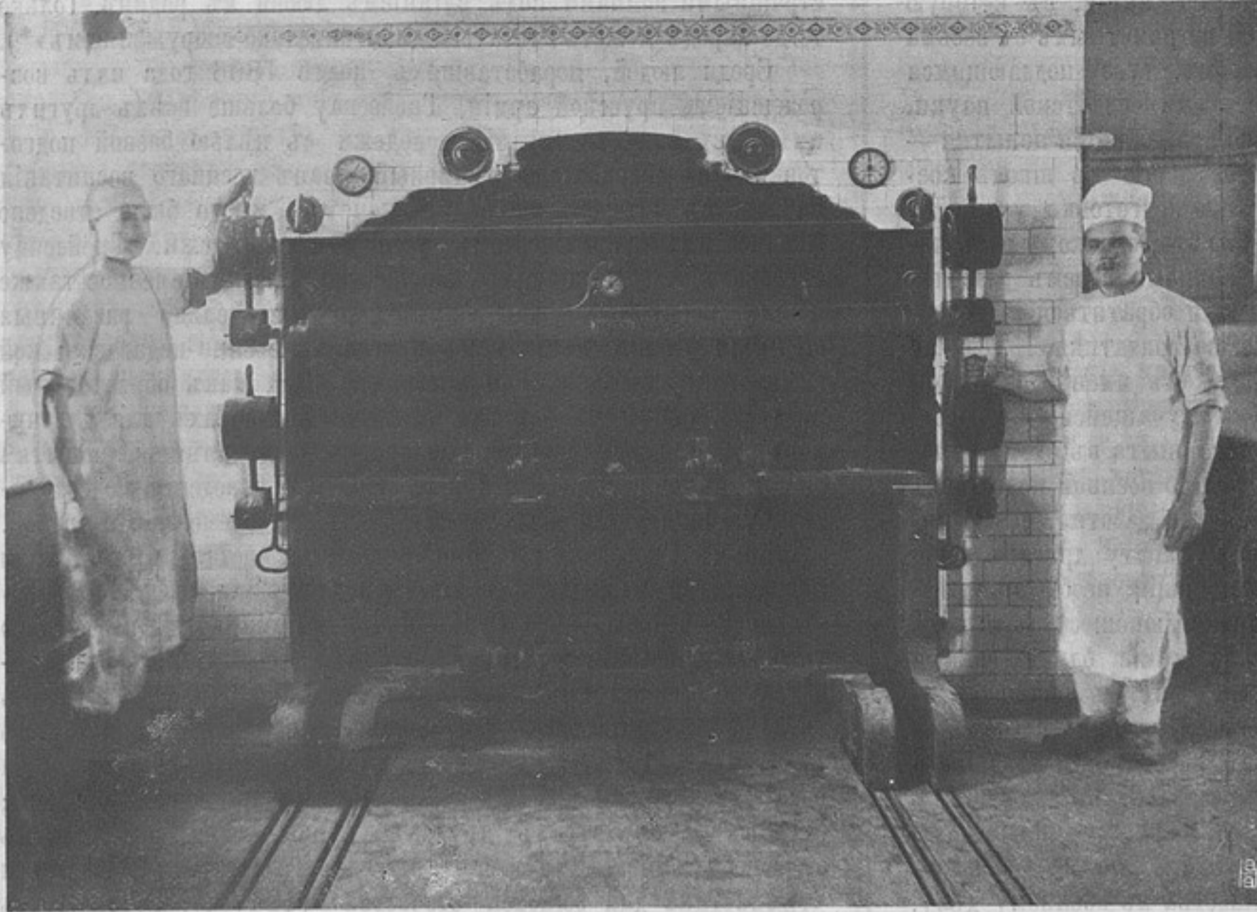
Наружный вид печи съ задвинутыми подами. (Къ ст. «Солдатскій хлѣбъ»).
