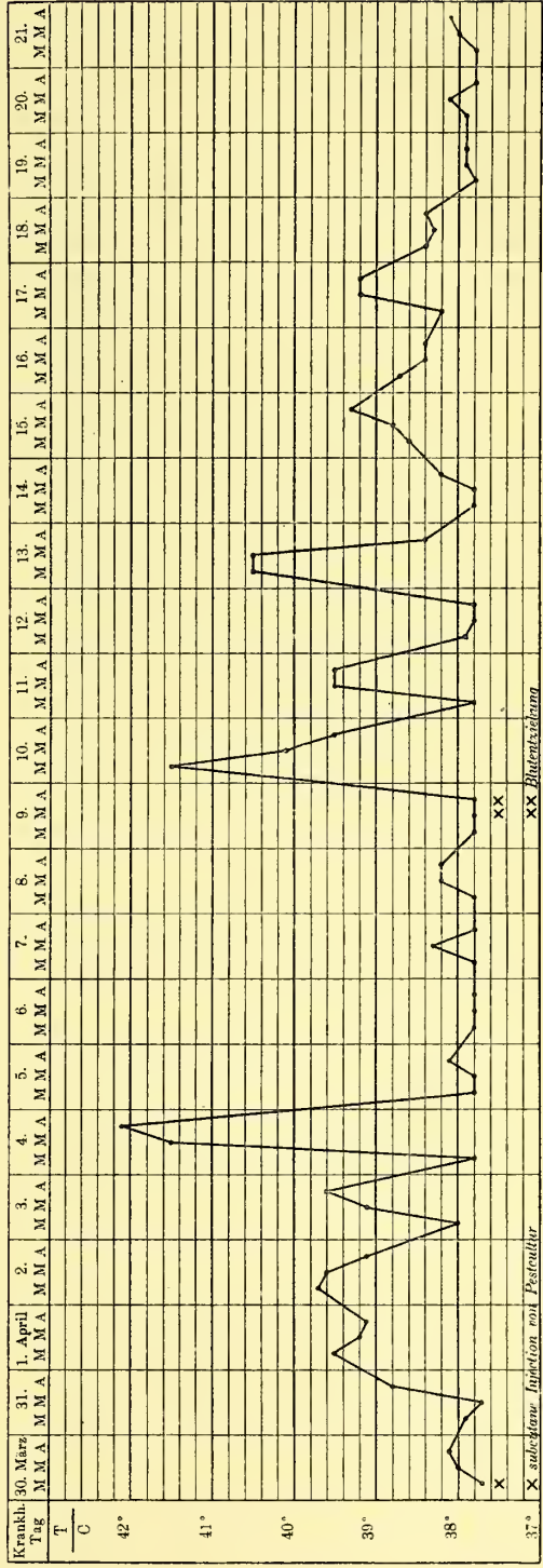
Temperaturkurve II.
