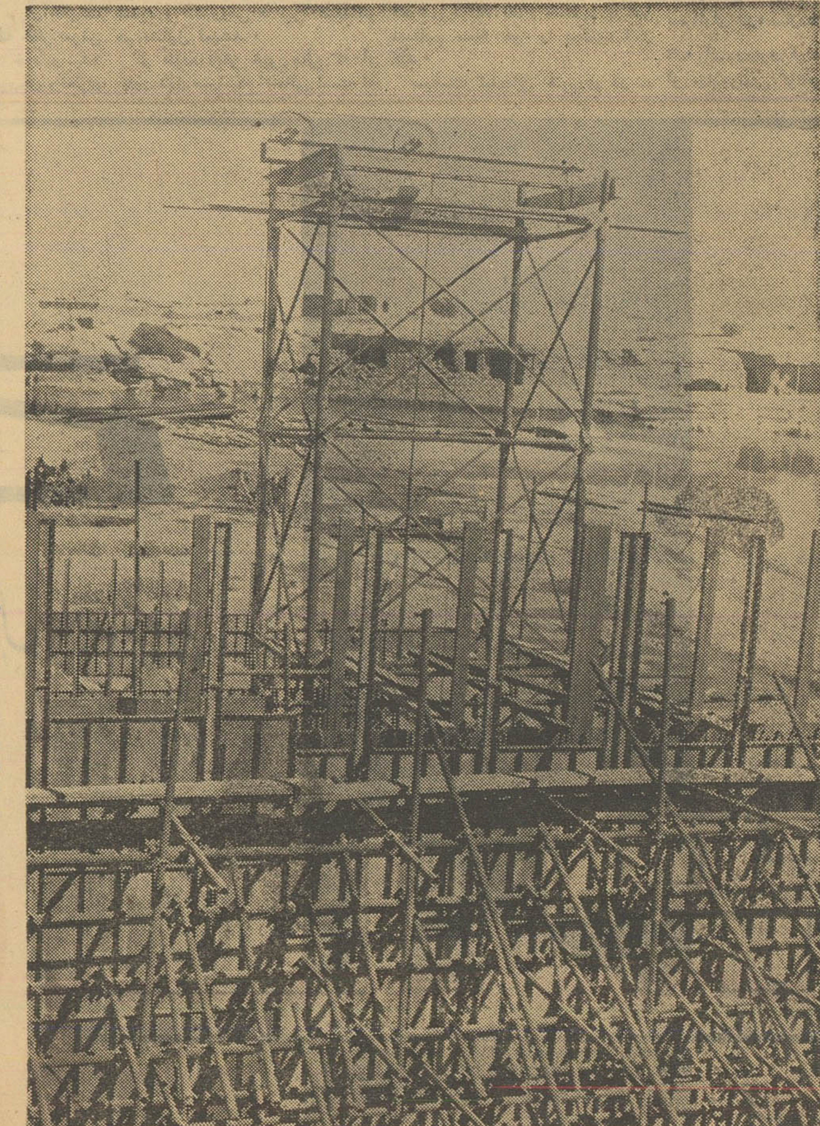
قسمتی از قالب بندیهاییکه بمنظور ریختن بتن در پایه ها بکار برده میشود
