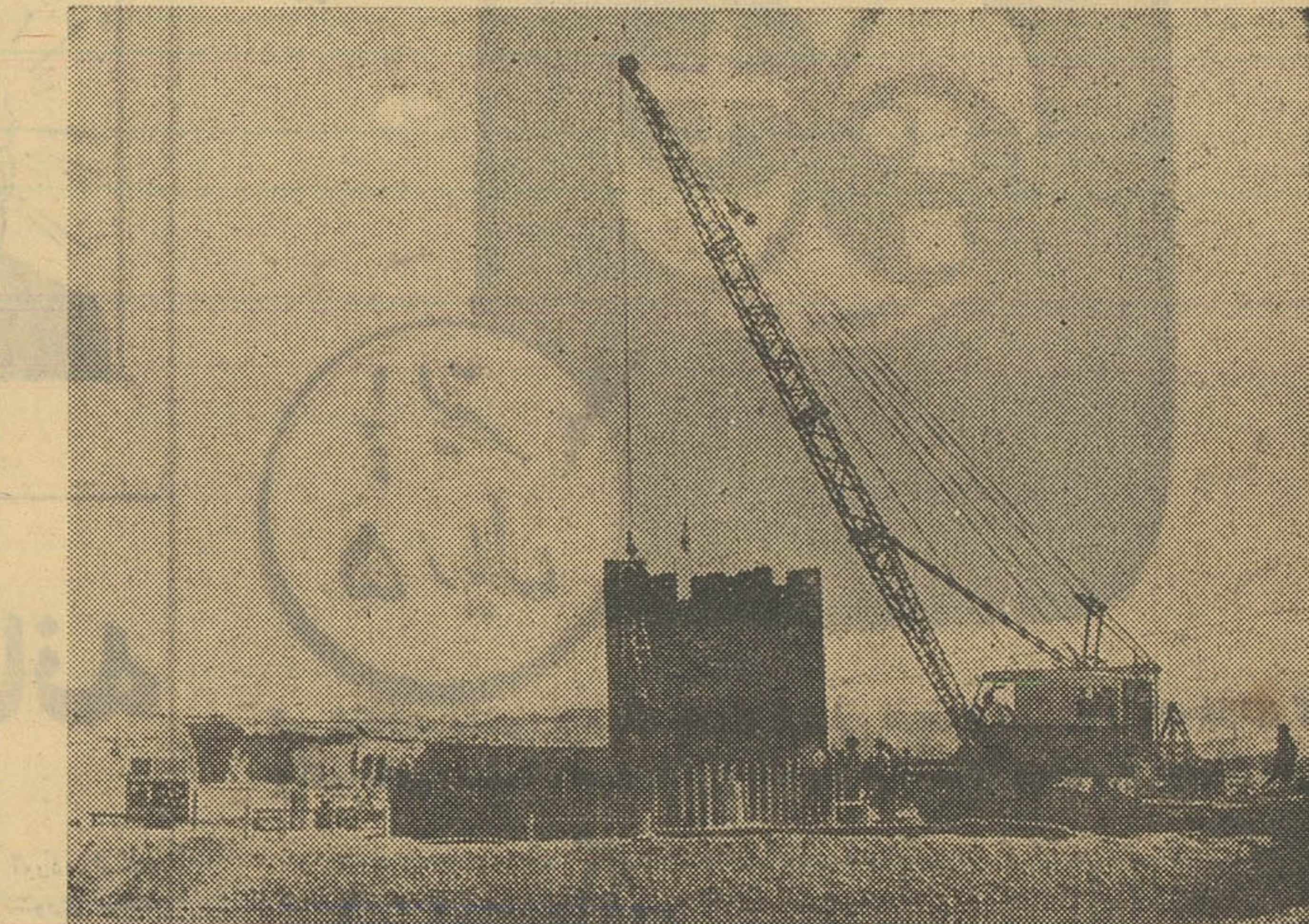
قسمت دیگری از پیل هایی که اکنون تا عمق ۱۵ متری در رودخانه فرو برده شده
