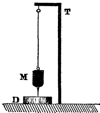
計動地之單簡最 圖八第
