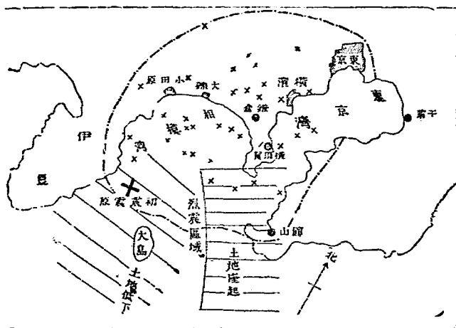
第五圖 最近日本地震區圖
