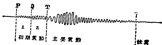
第十圖 地震波圖之範圍
