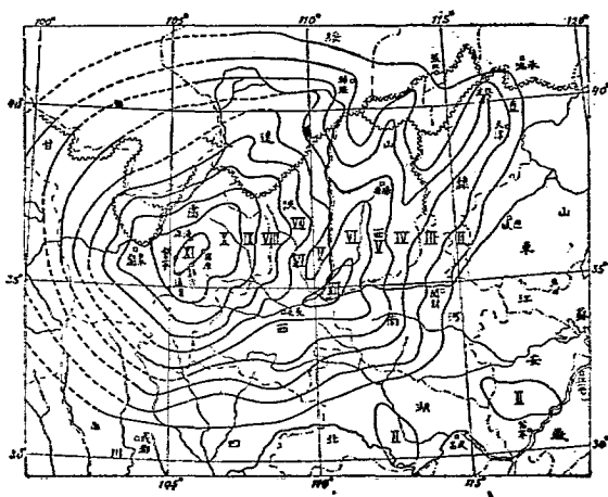
圖震地肅甘年九國民 圖六第
