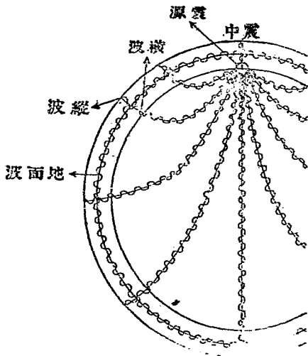
第十圖 地震波之傳播
