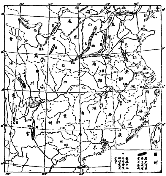
圖布分區中震地國中 圖五十第
