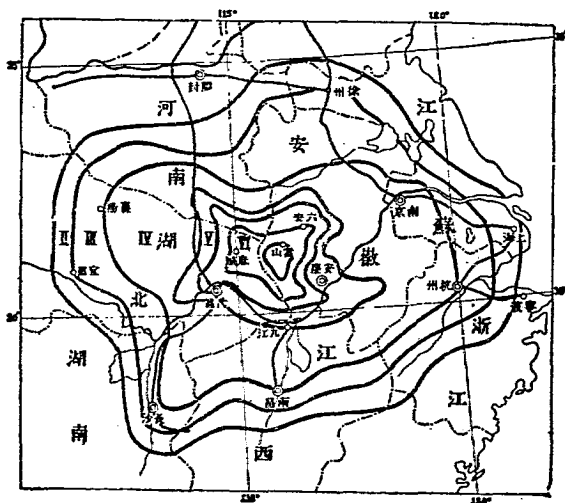
圖震地徽安年六國民 圖六十第
