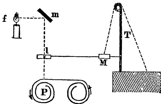
種一之計動地 圖九第
