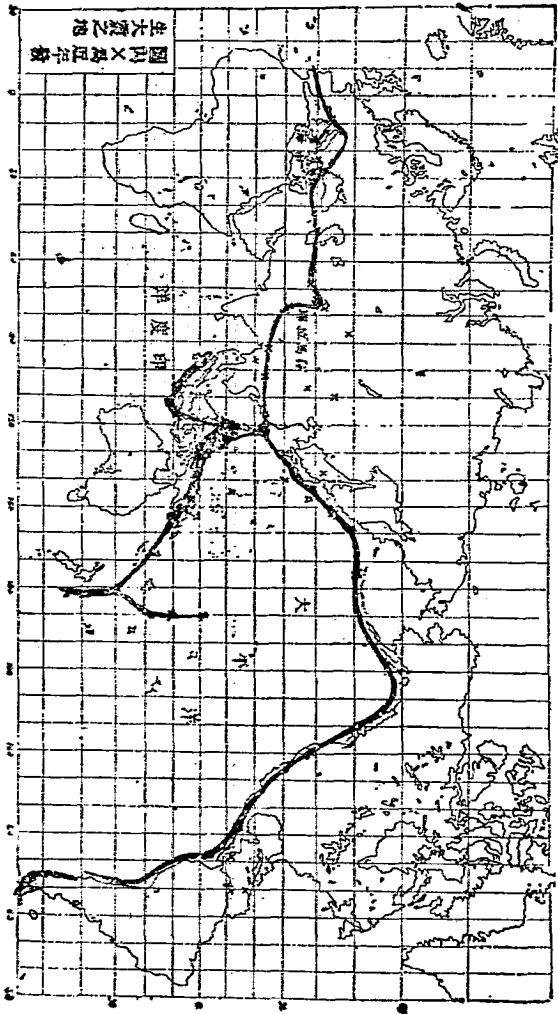
圖 三 十 第 大 平 洋 周 圍 中 地 海 分 佈 圖
