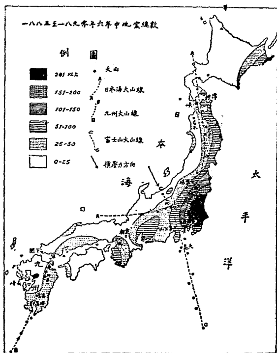
圖布分震地本日本 圖四第十
