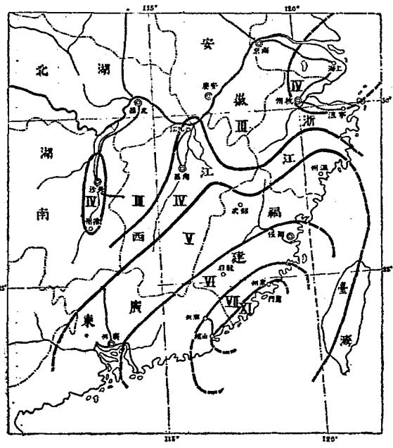
圖七十第 國民七年福建地震圖
