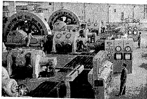
我國自己設計、製造設備和施工安裝的 大型肥料機——廣州氮肥廠，最近正式投入生 產。這台機器，合成氣車間，(新華社記者孔繁根攝)
