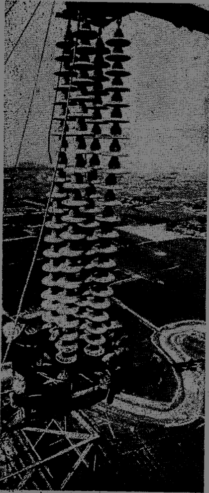
上海市供电局高压工区工人在浦东农村上空，检修高压线路，使电力源源供应农村，支援春耕生产。 (新华社记者唐允仁摄)
